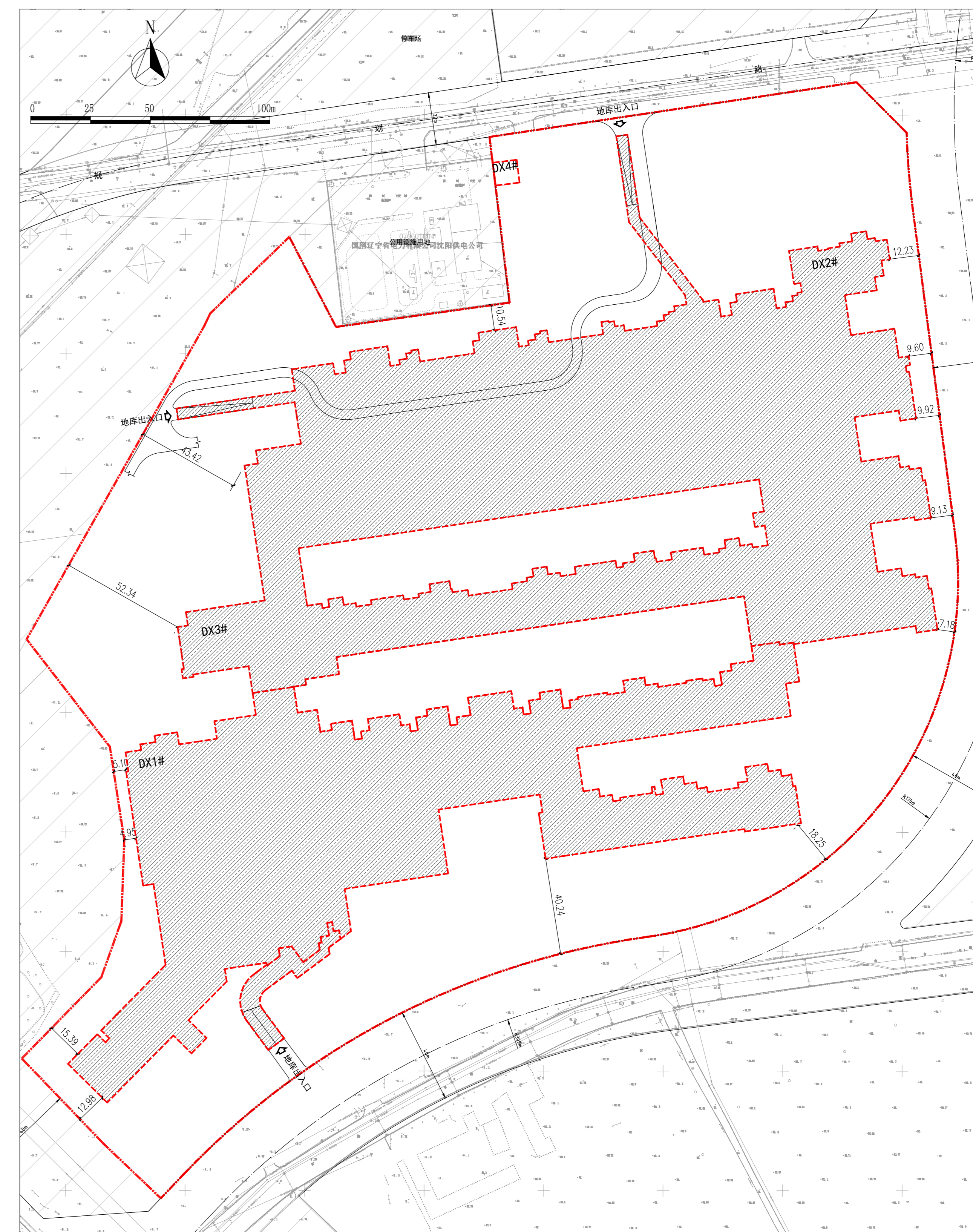
变更后总平面图
