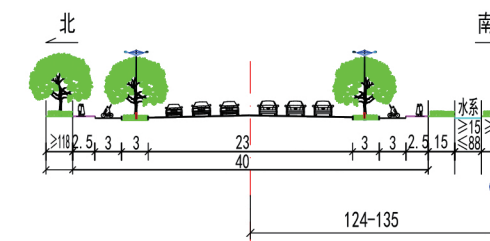
白塔河路规划横断面
