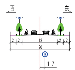
白塔三街规划横断面
