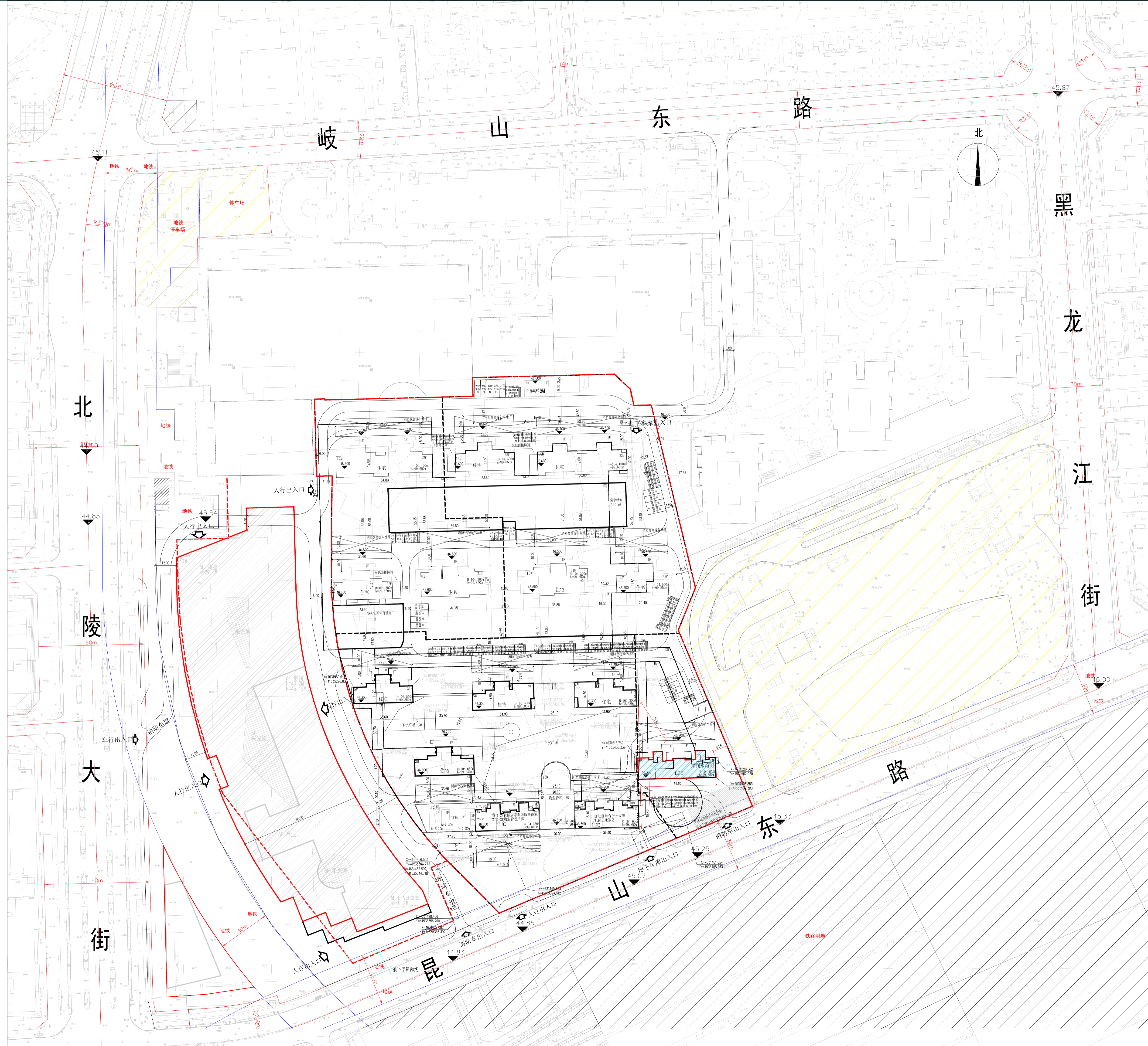
总平面图1:1000
