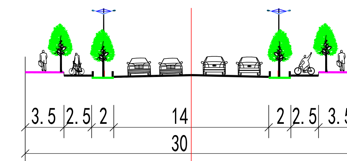
2号路道路规划横断面
