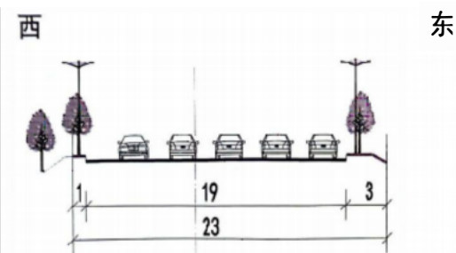
青年大街-远航路匝道规划横断面
