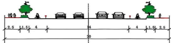
清泉路道路规划横断面
