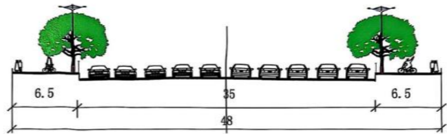
大北关街道路规划横断面
