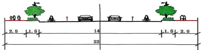
甘泉路道路规划横断面
