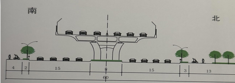
东北大马路道路规划横断面
