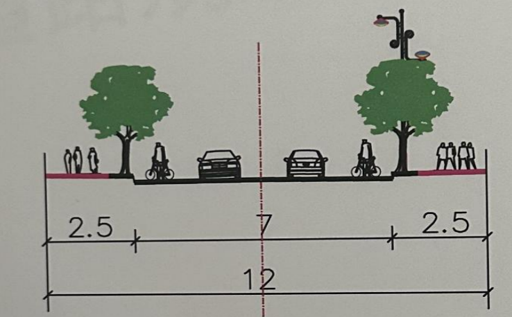
钢泉巷道路规划横断面
