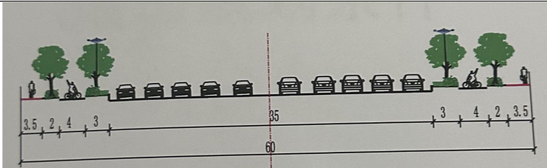
东望街道路横断面规划
