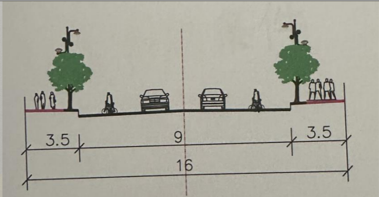
钢泉巷道路规划横断面
