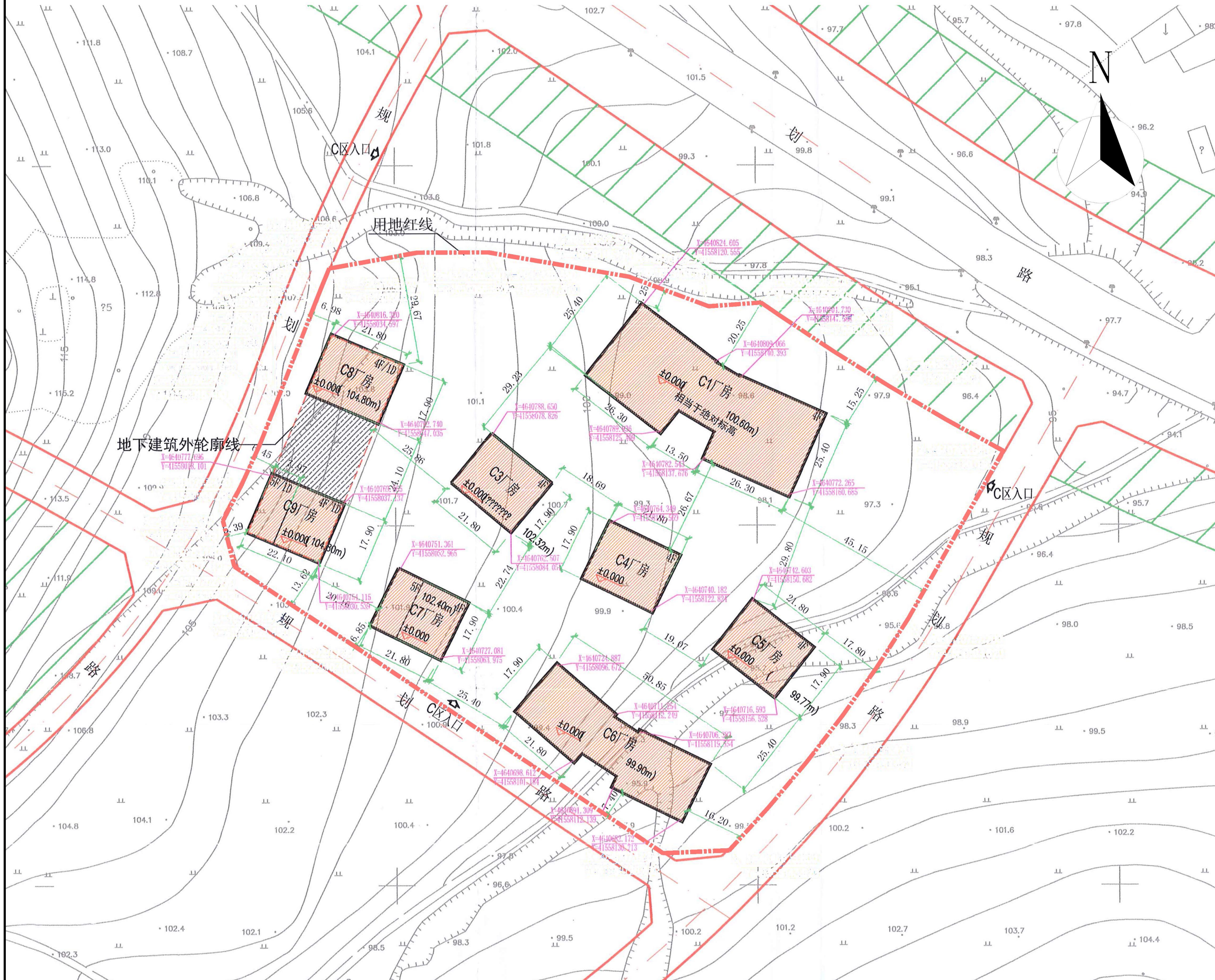
变更前总平面图
