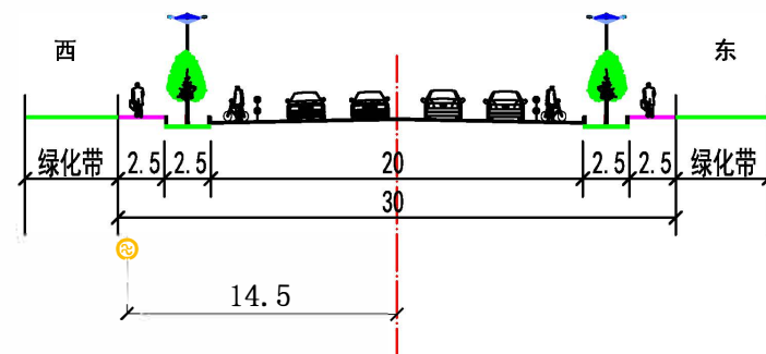
上深沟街(双深路~美食美刻) 规划横断面
