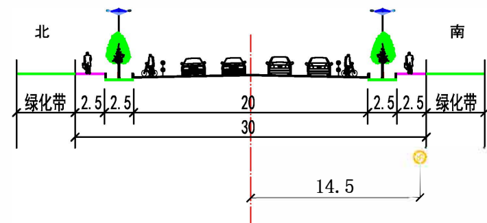
双深路(沈本一街~上深沟街) 规划横断面
