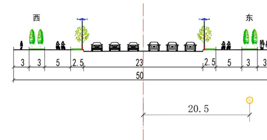
朗日街规划横断面
