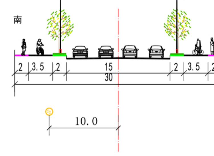
银卡路规划横断面
