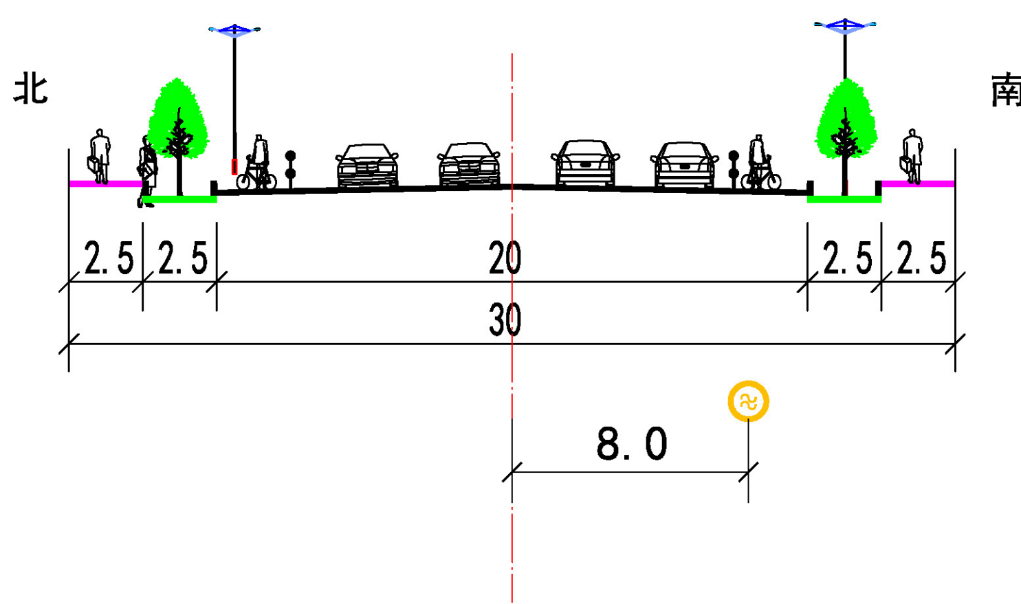
三环南三路规划横断面
