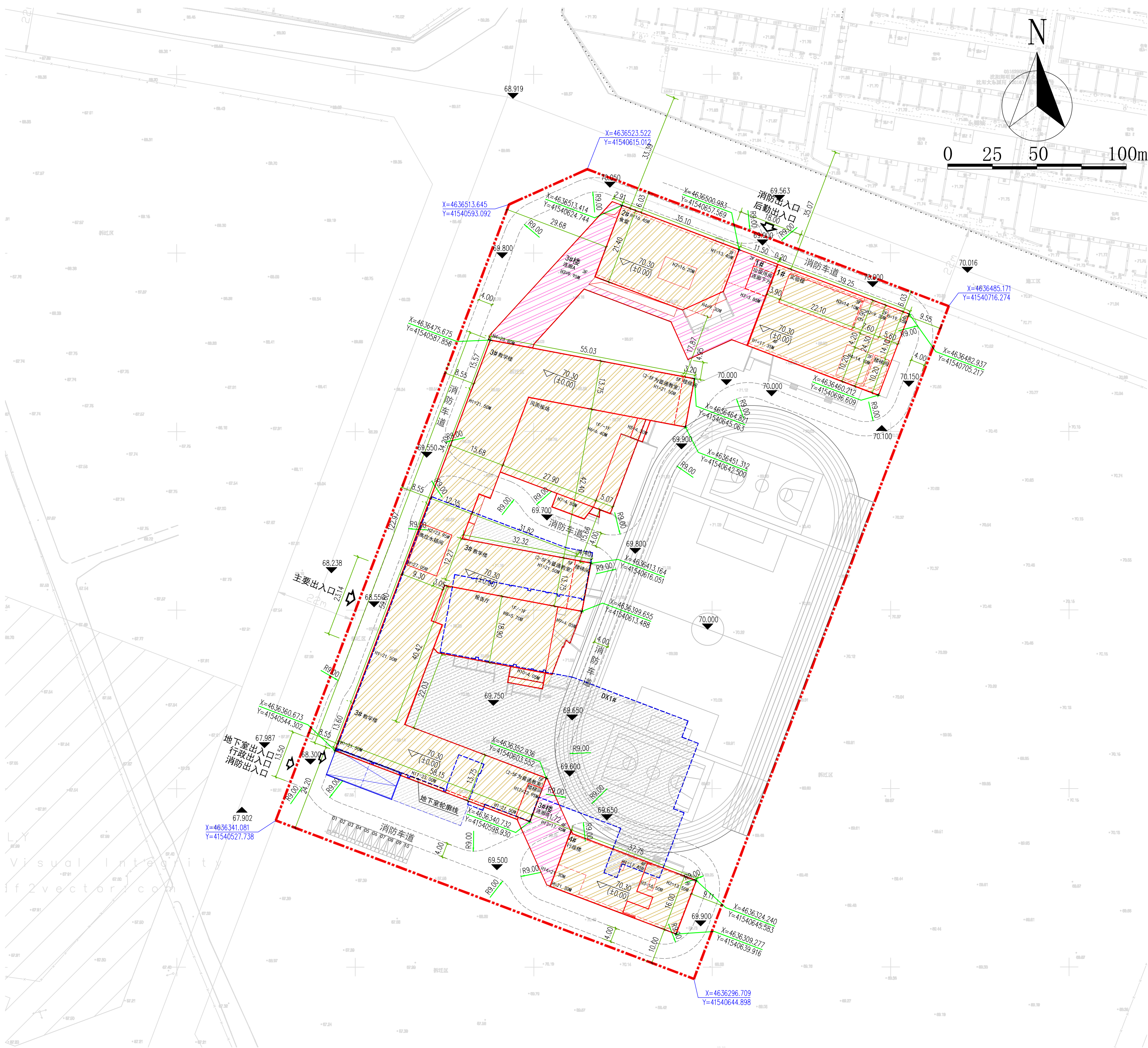
规划设计方案总平面图
