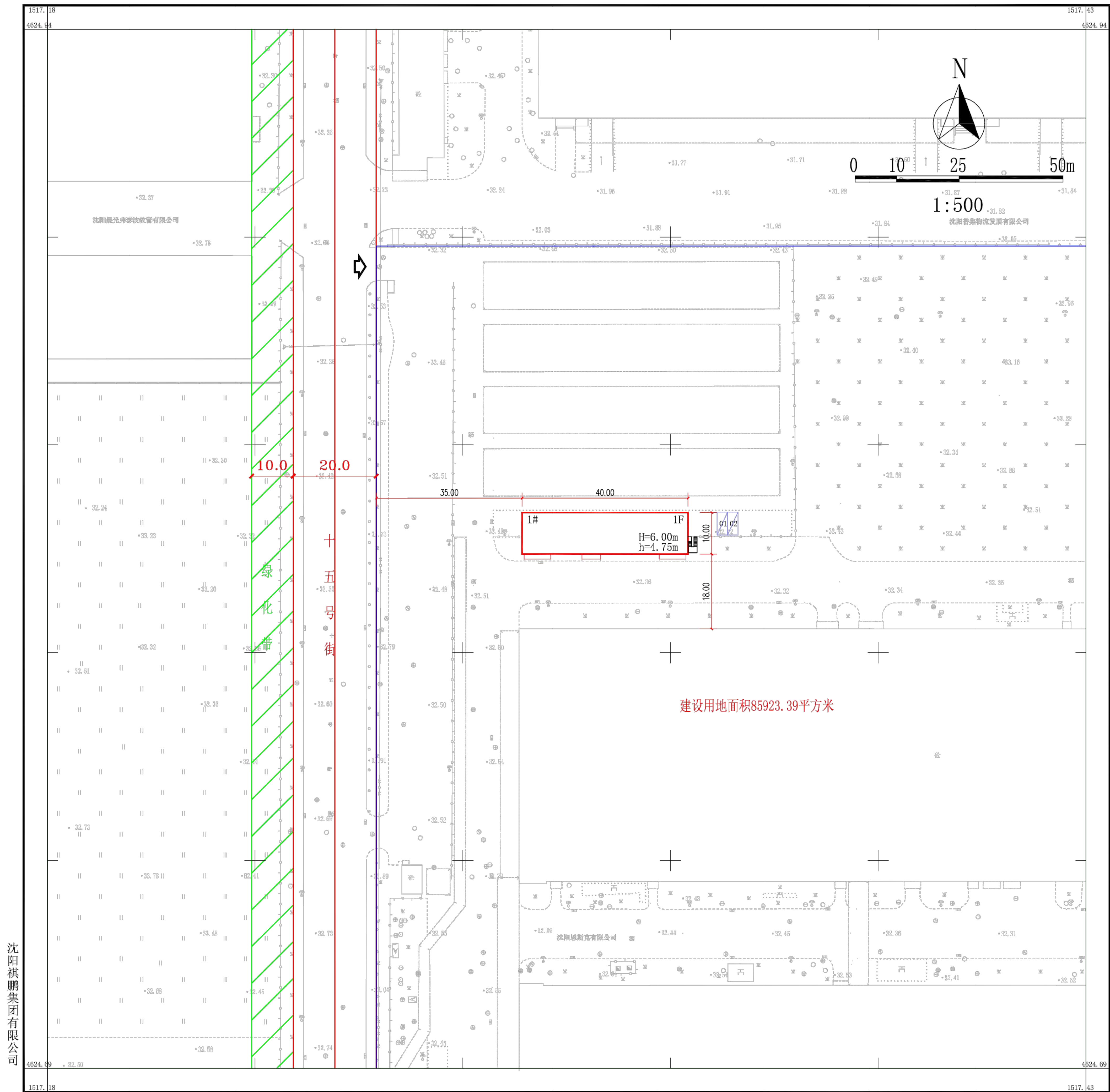
建设工程规划许可证附图
