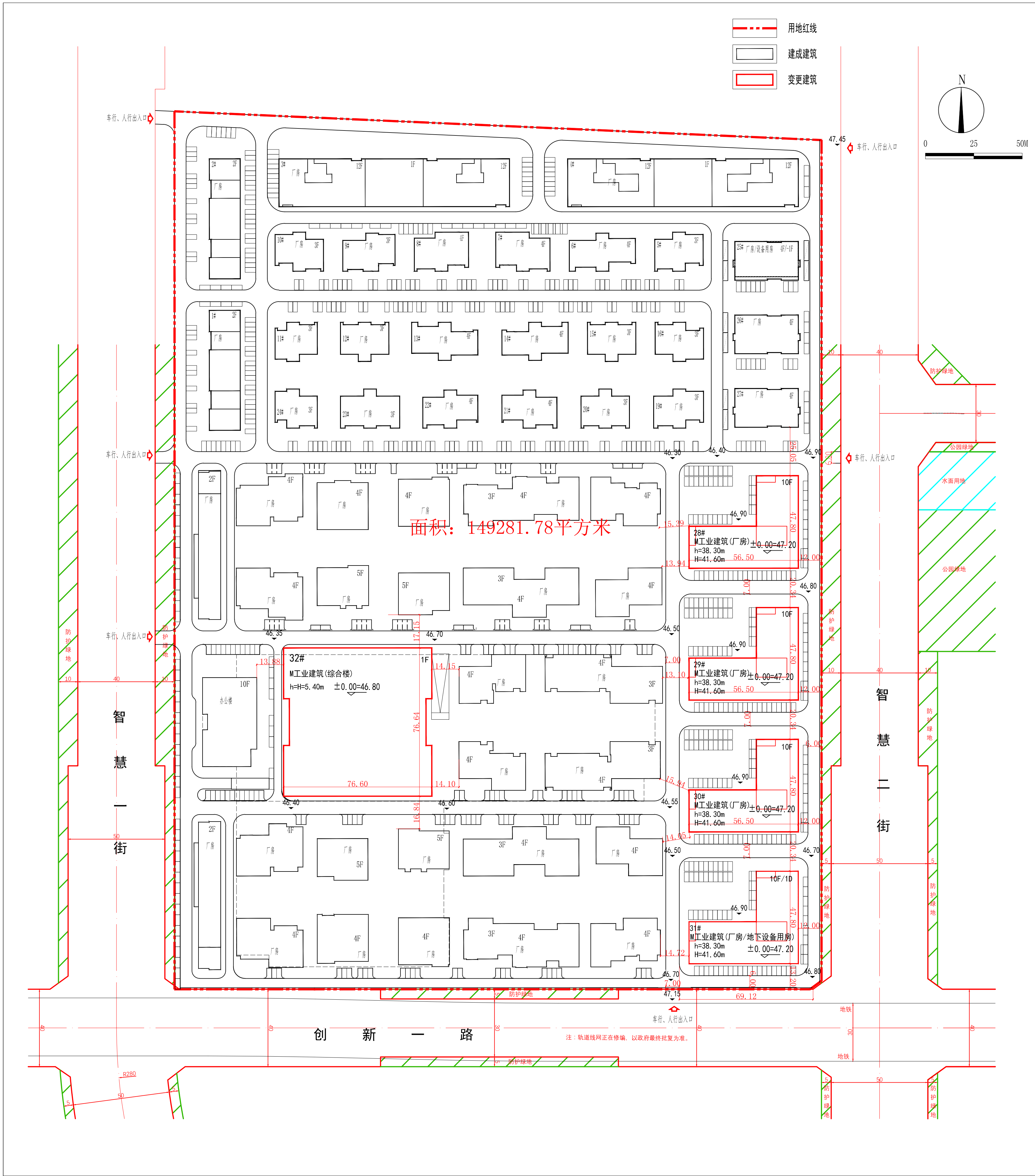
变更后总平面图
