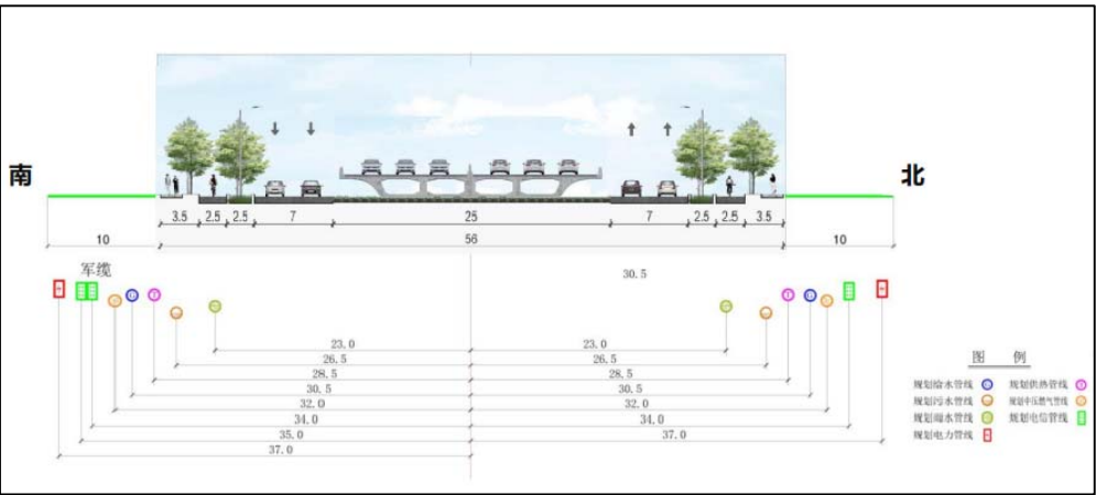
开发十八号路（浑河二街-浑河三街）电信项目 综合断面图
