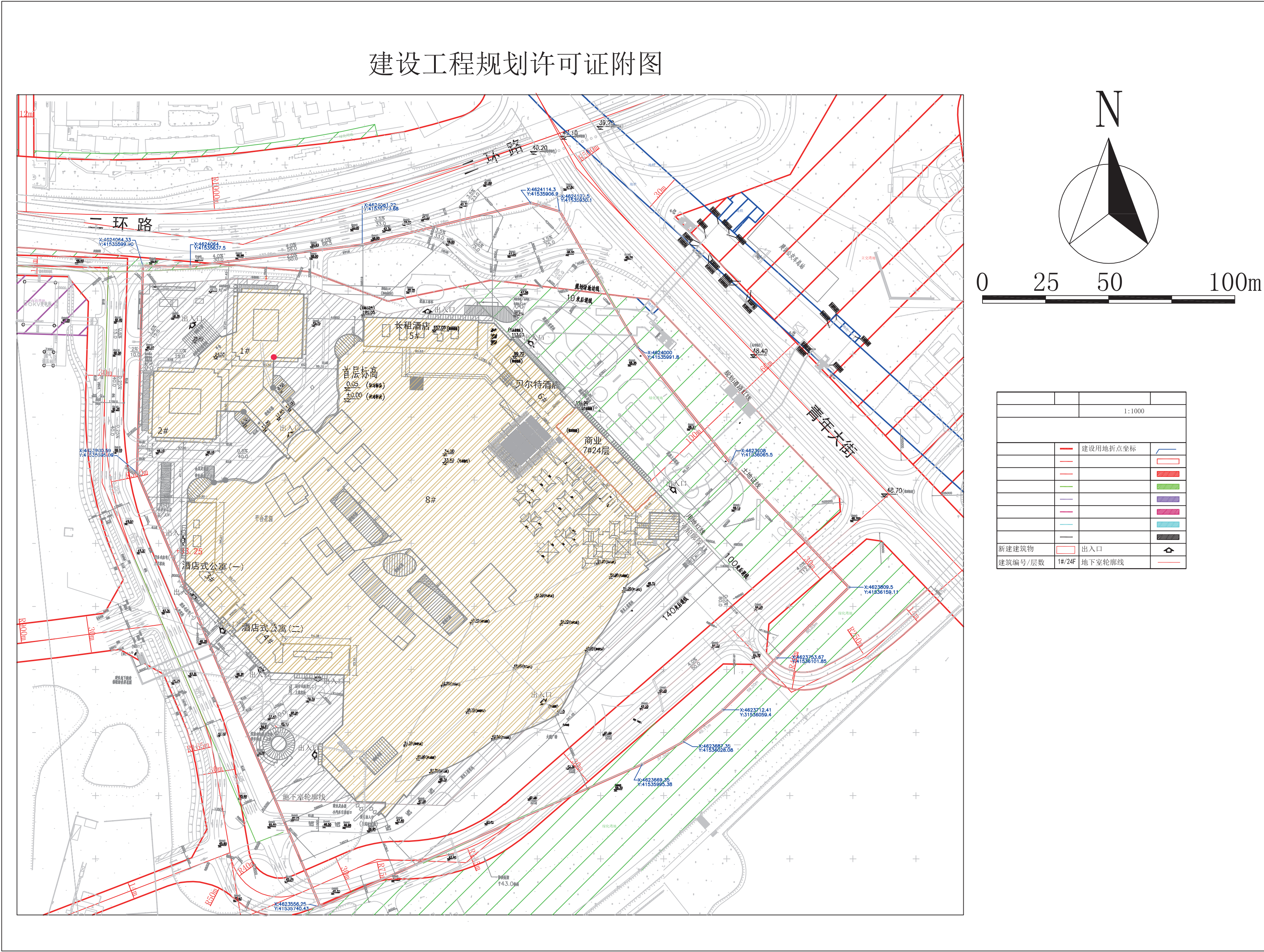
变更前总平面图
