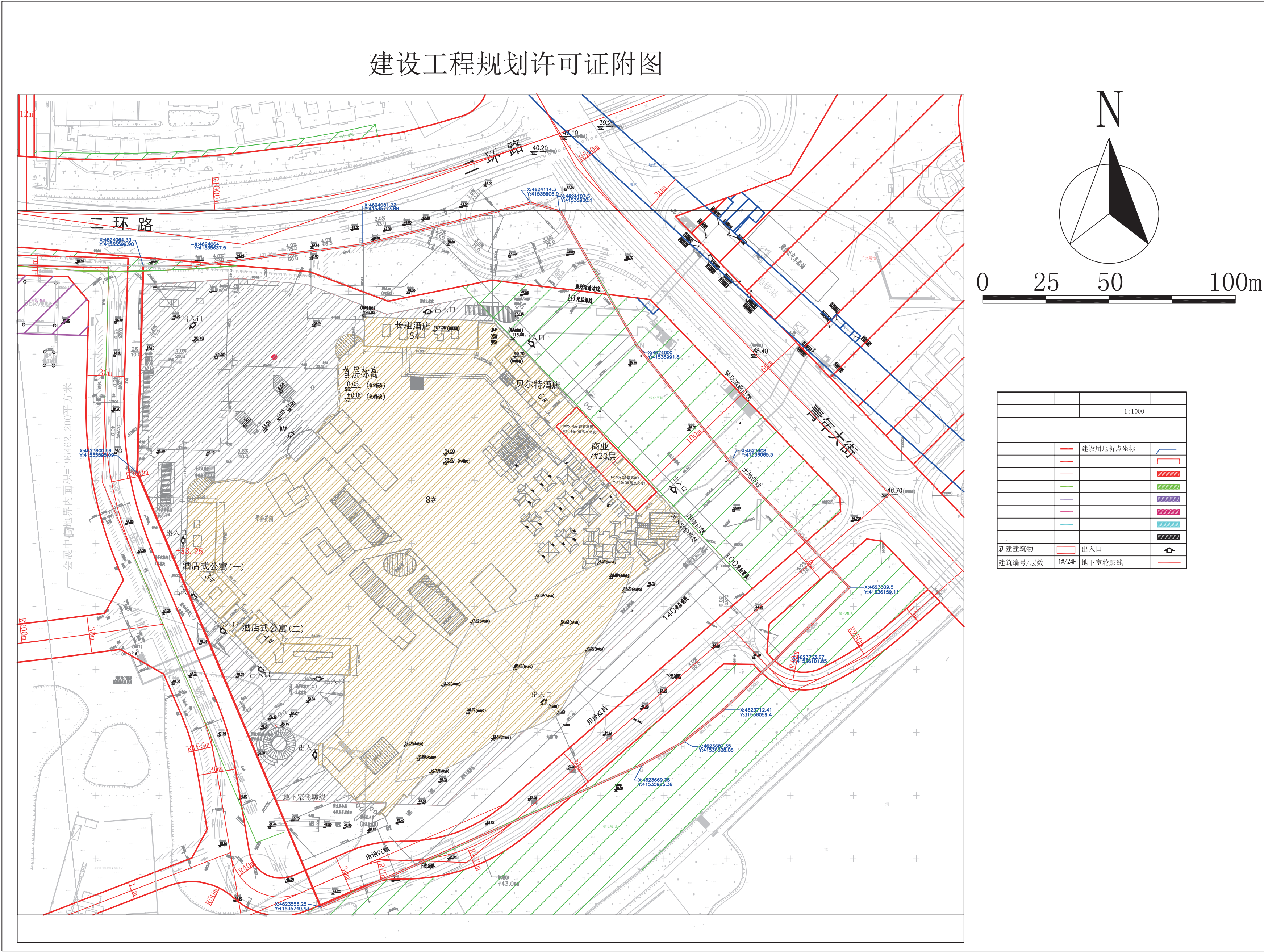
变更后总平面图
