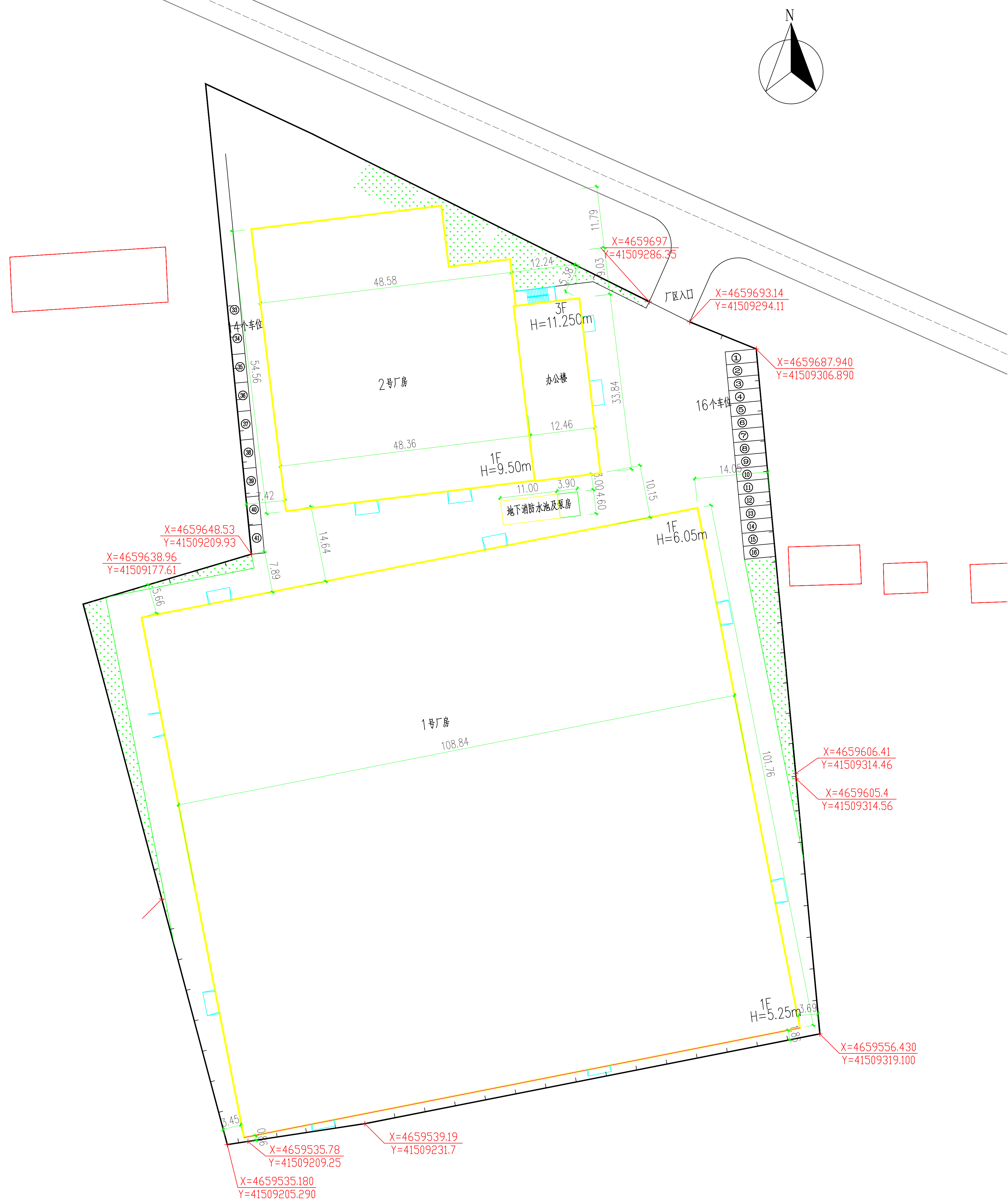
总平面布置图1:500
