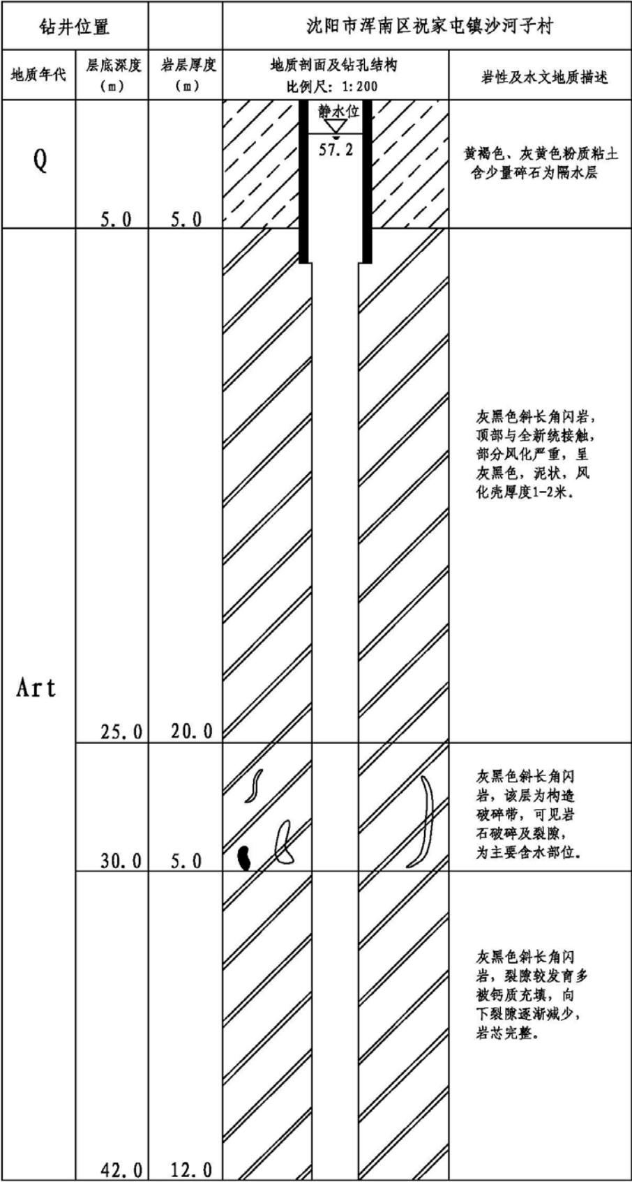
图 2-2 矿泉井柱状图
