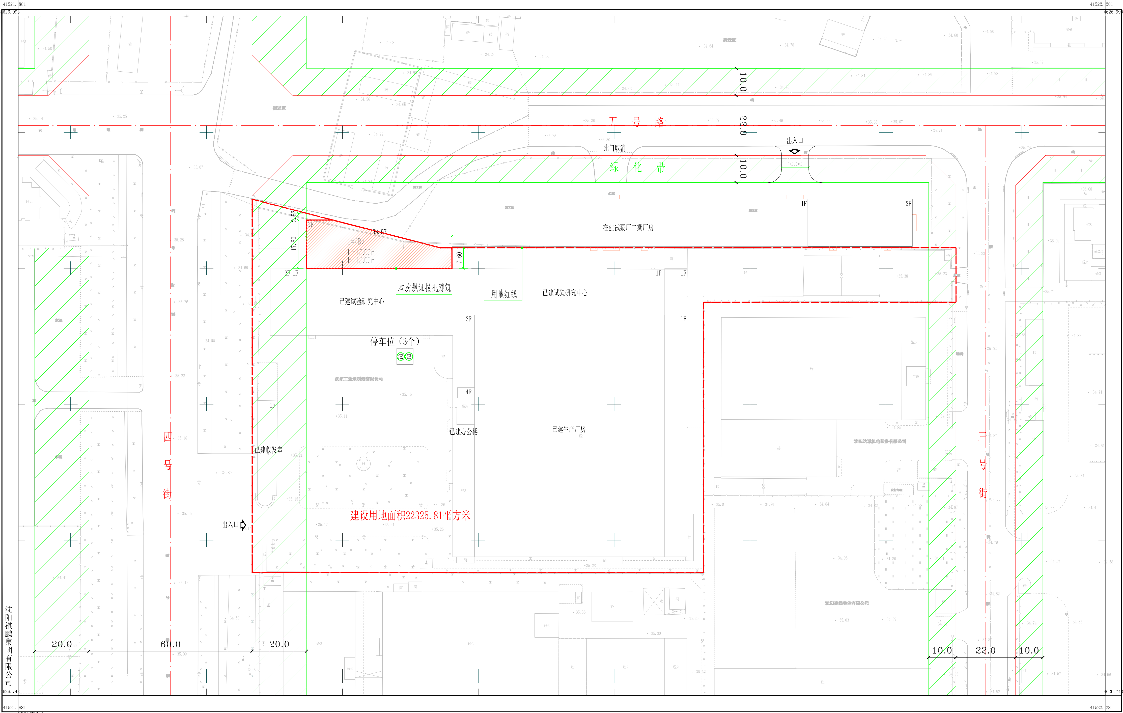
建设工程规划许可证附图
