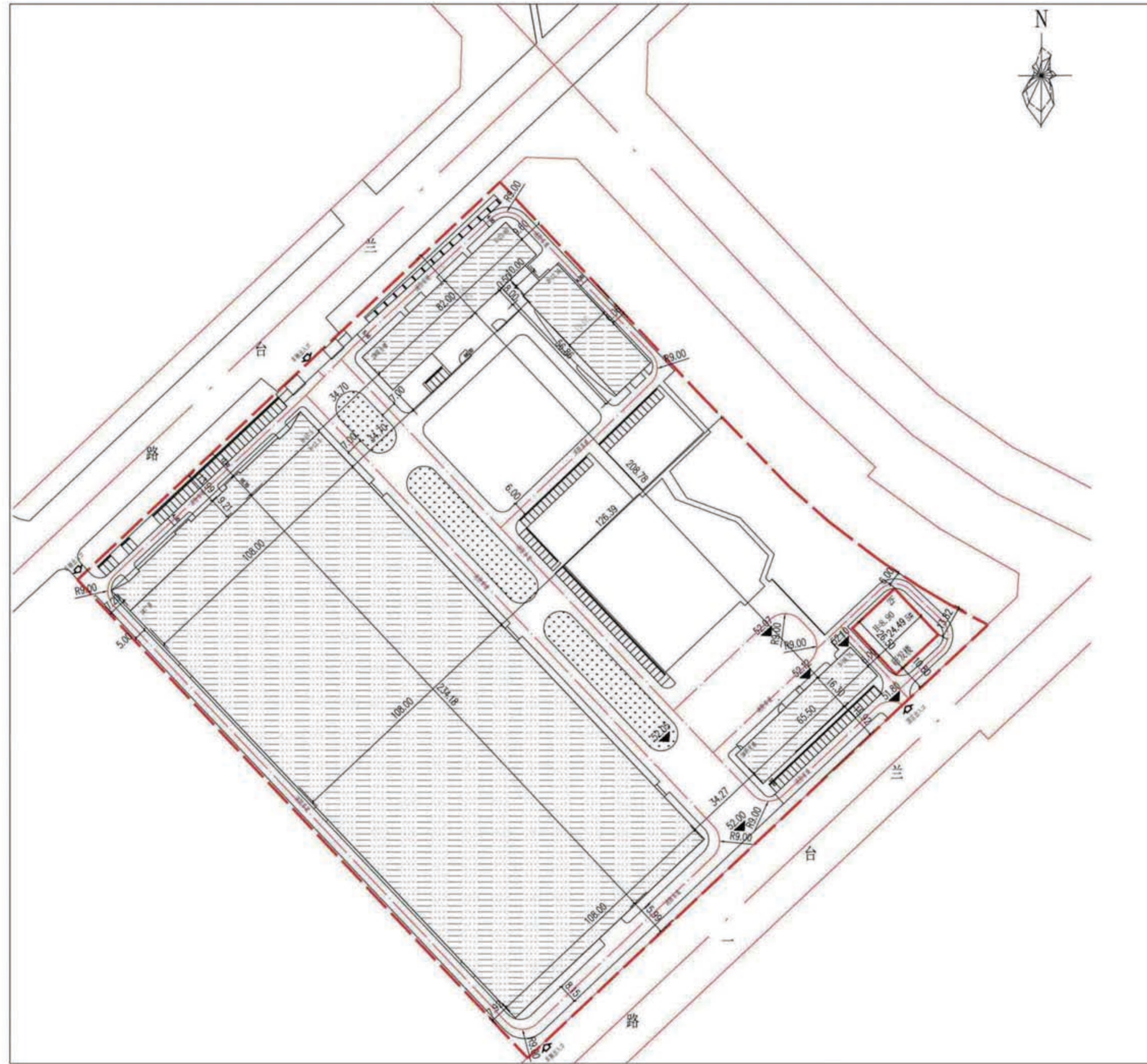
变更前总平面图
