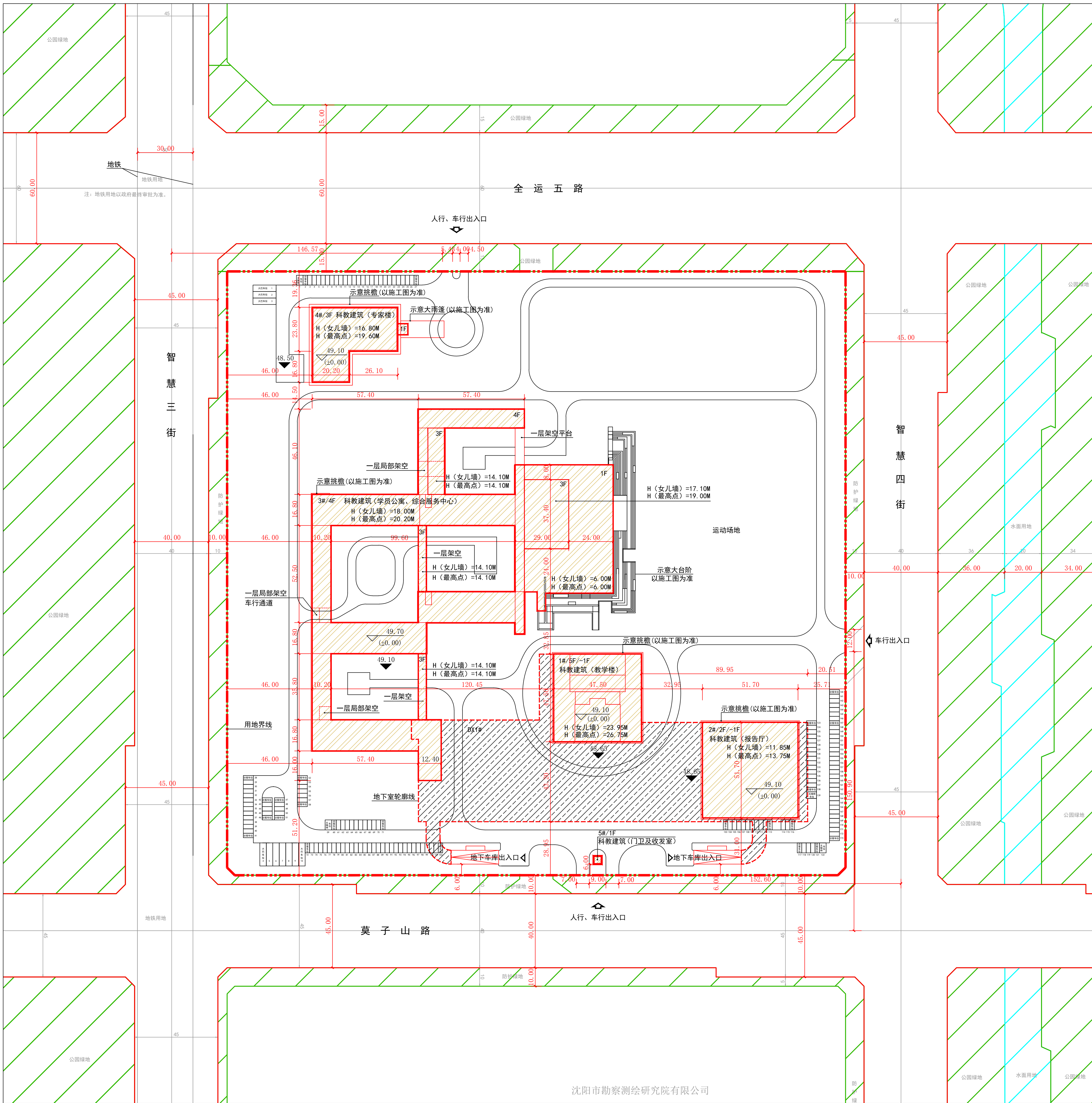
规划设计方案总平面图
