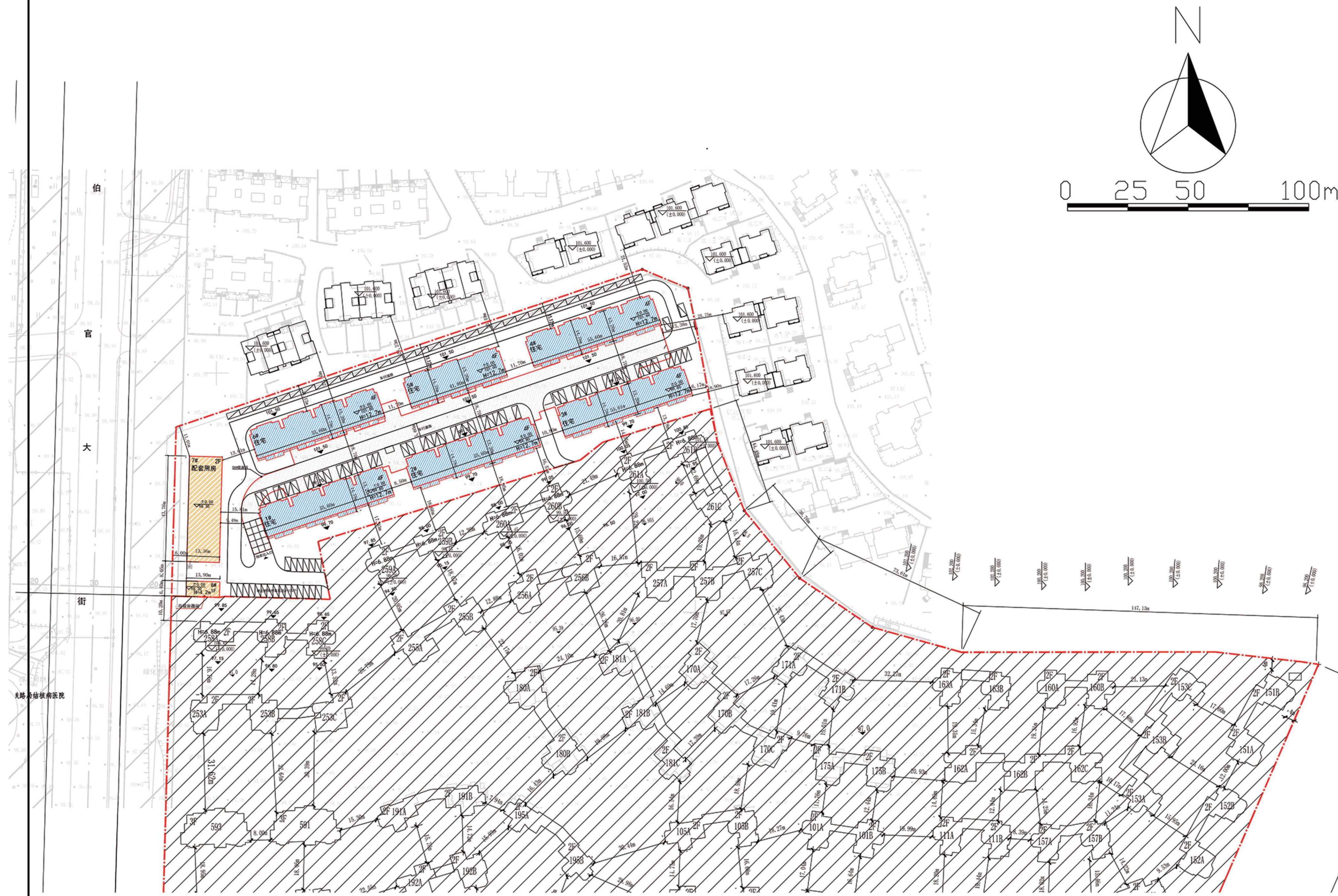
变更前总平面图
