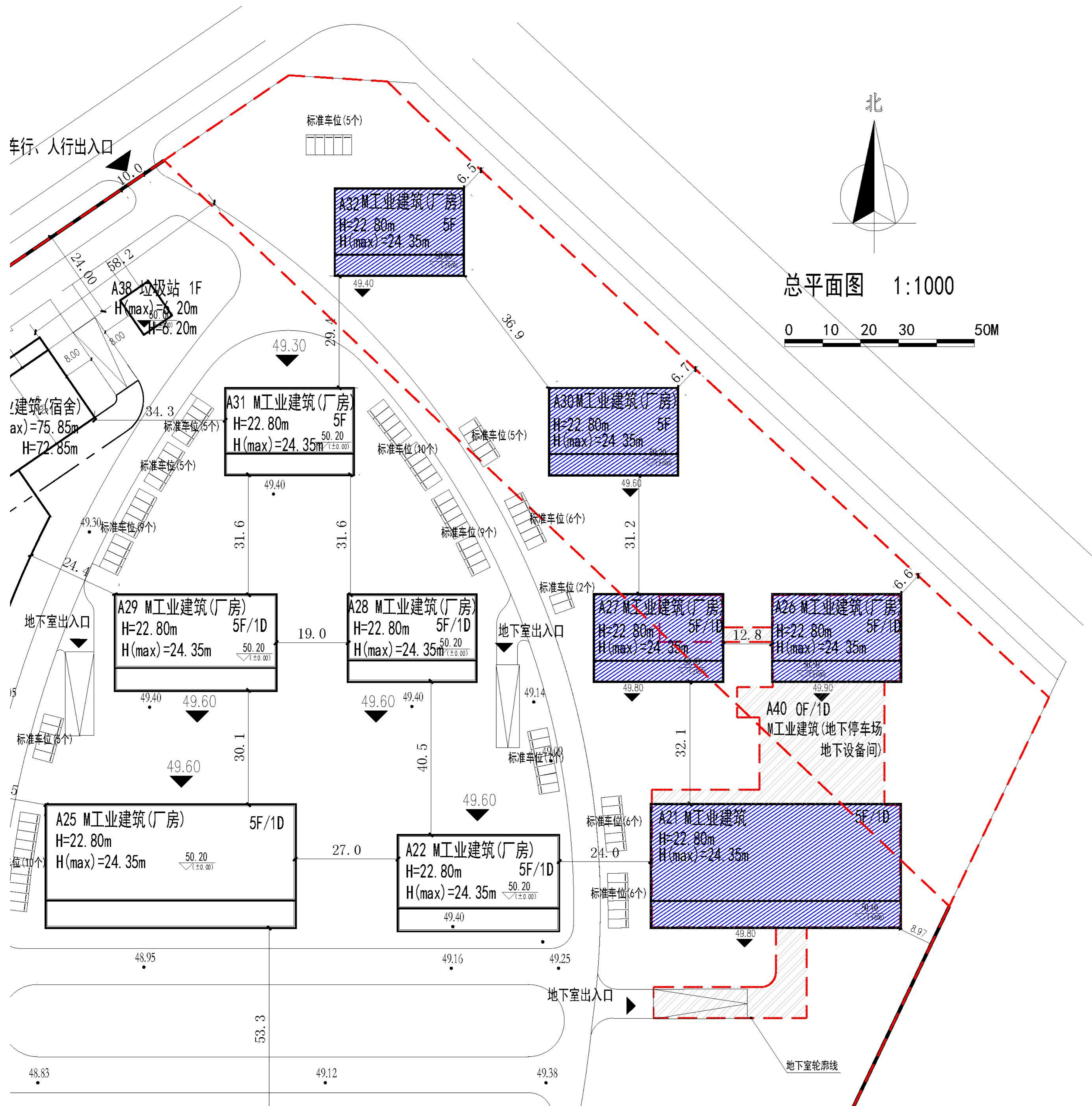
规划设计方案总平面图
