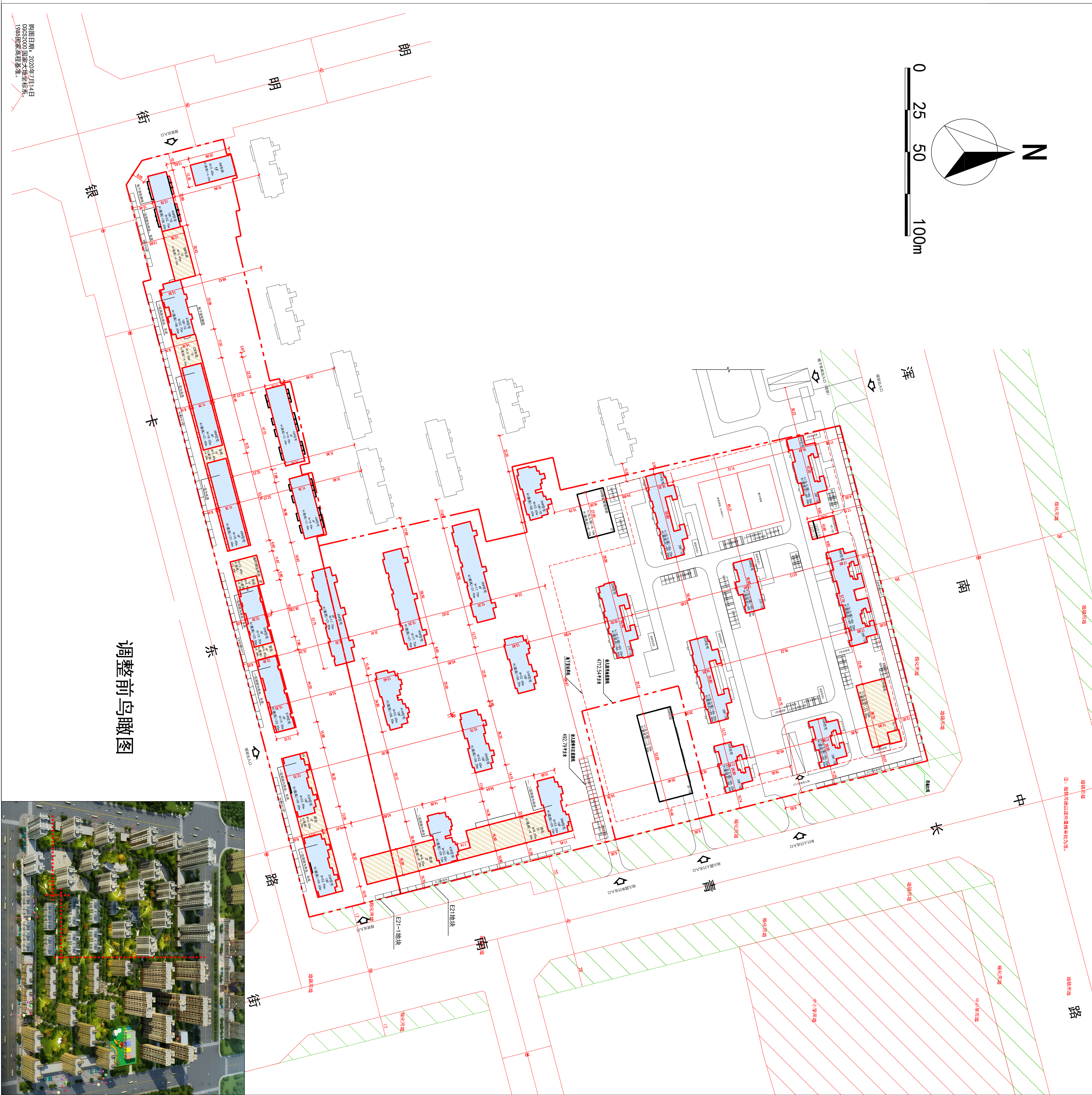
变更前总平面图
