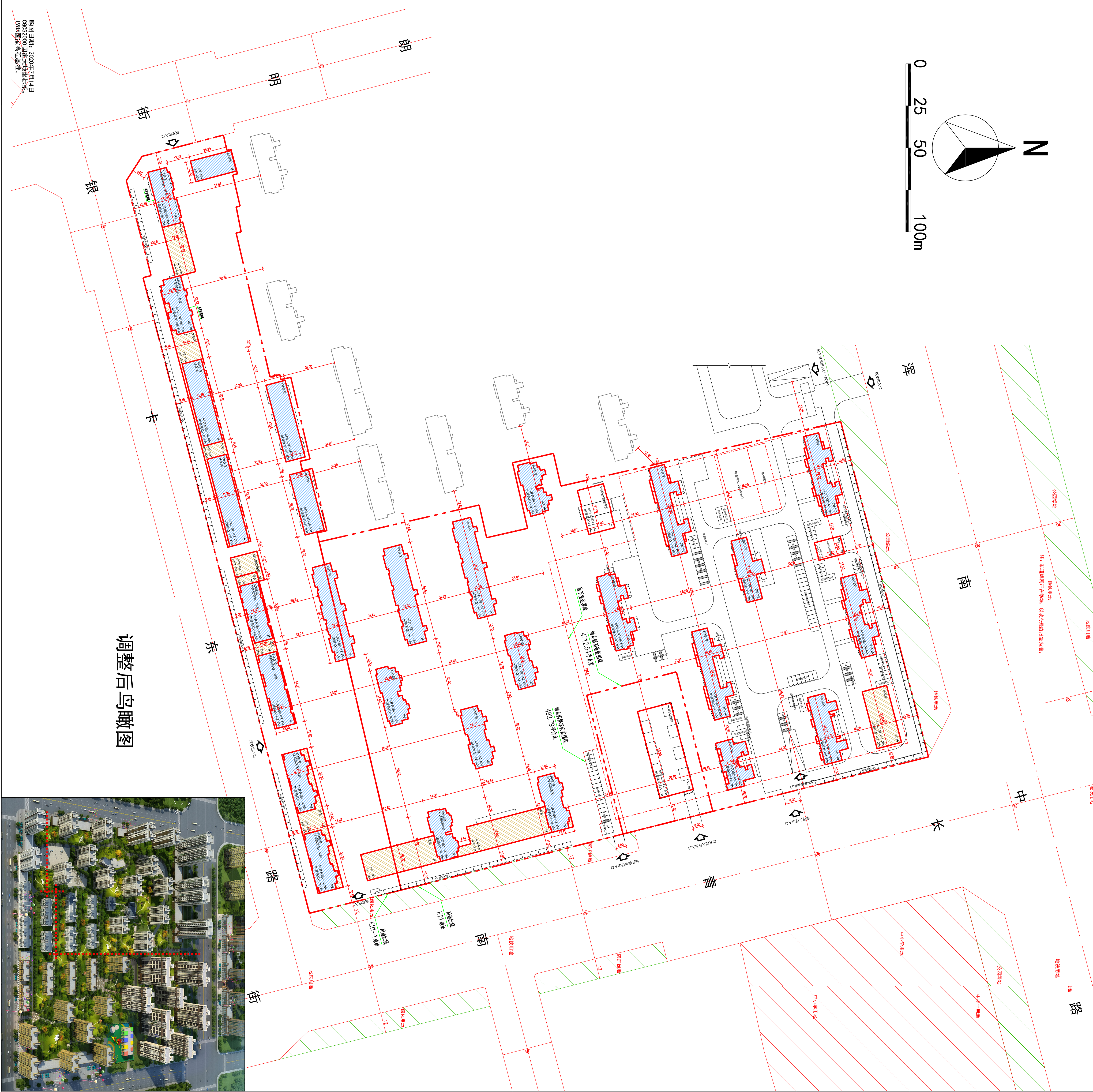
变更后总平面图
