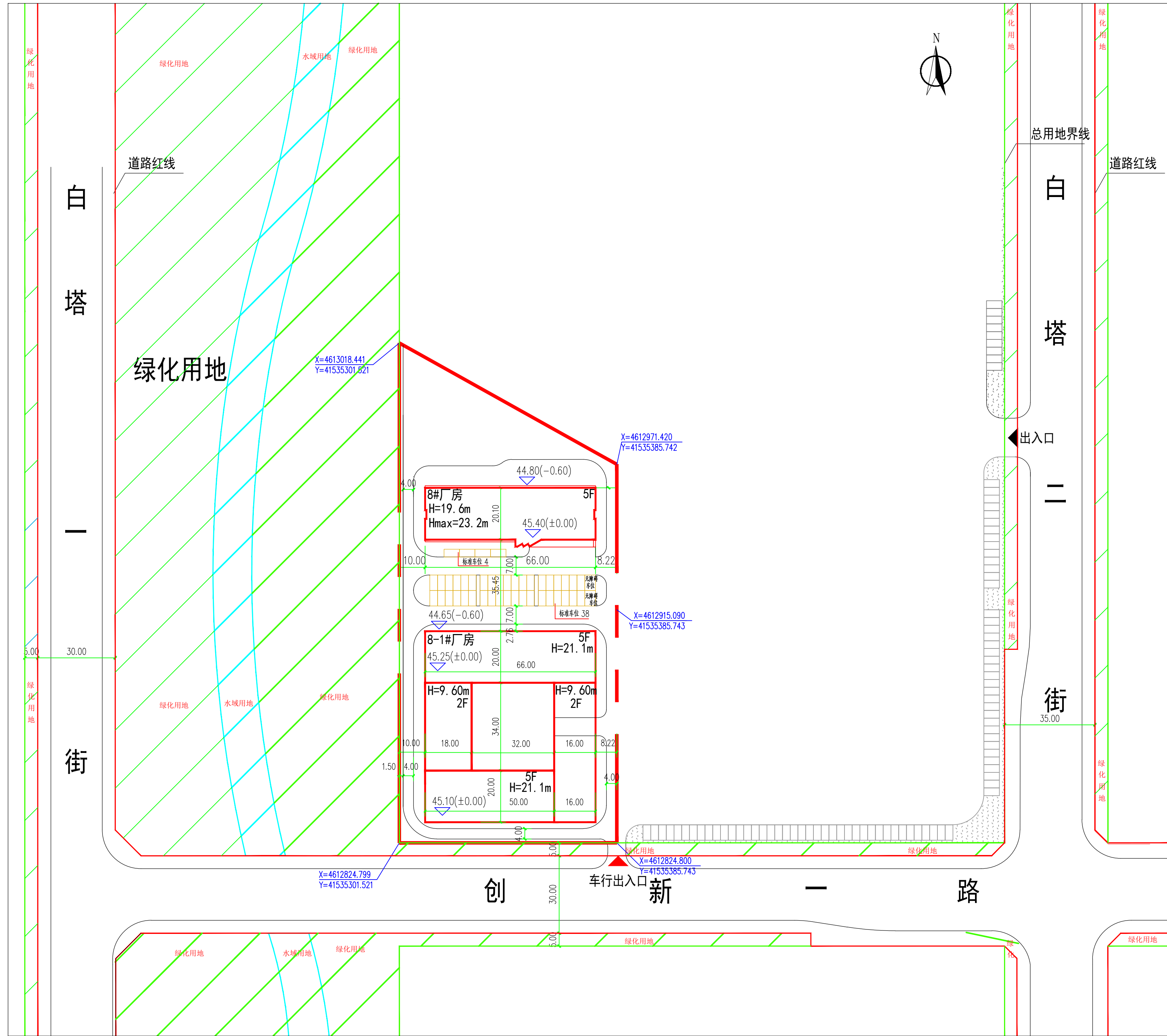
变更后总平面图
