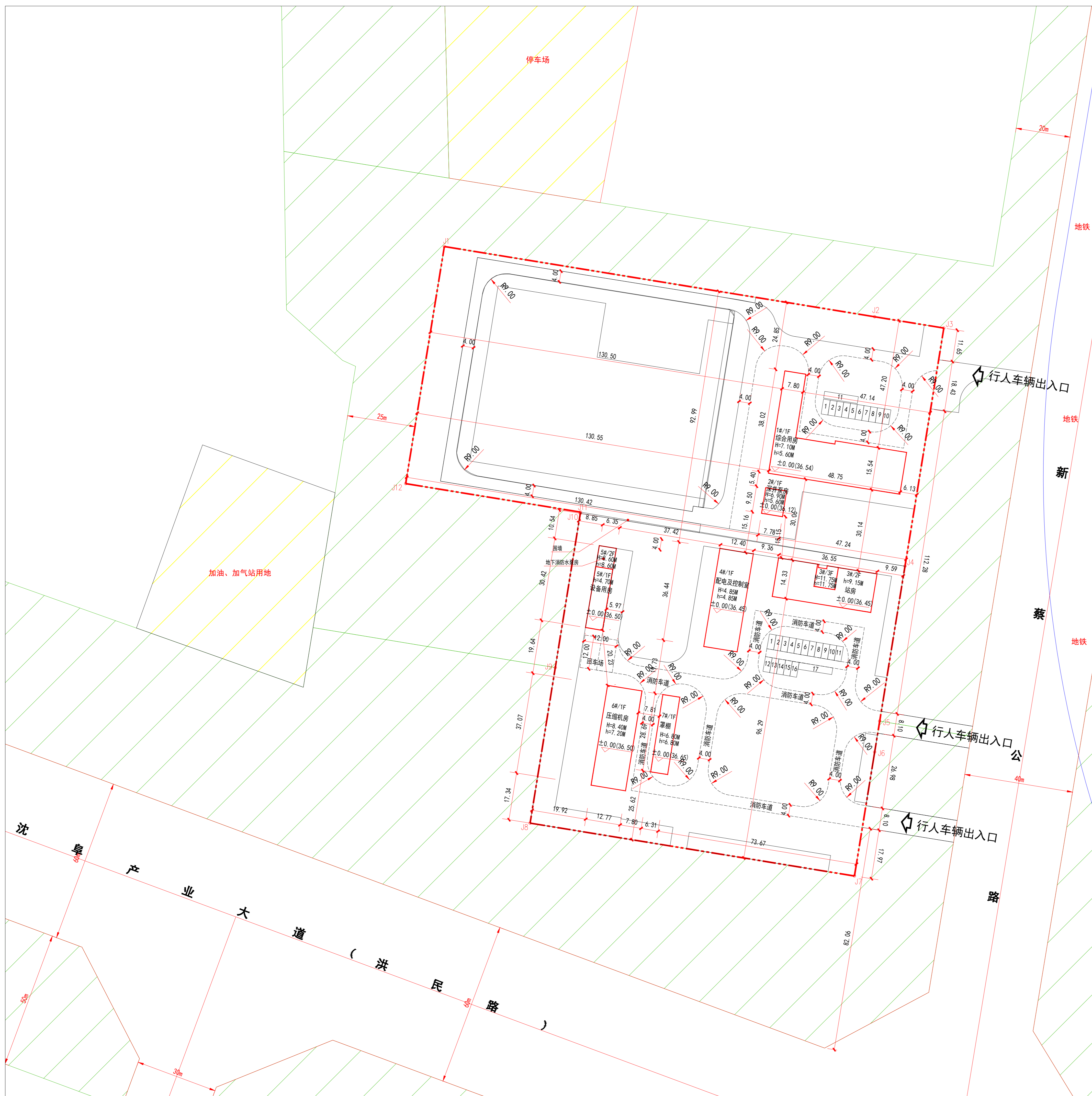
规划总平面图
