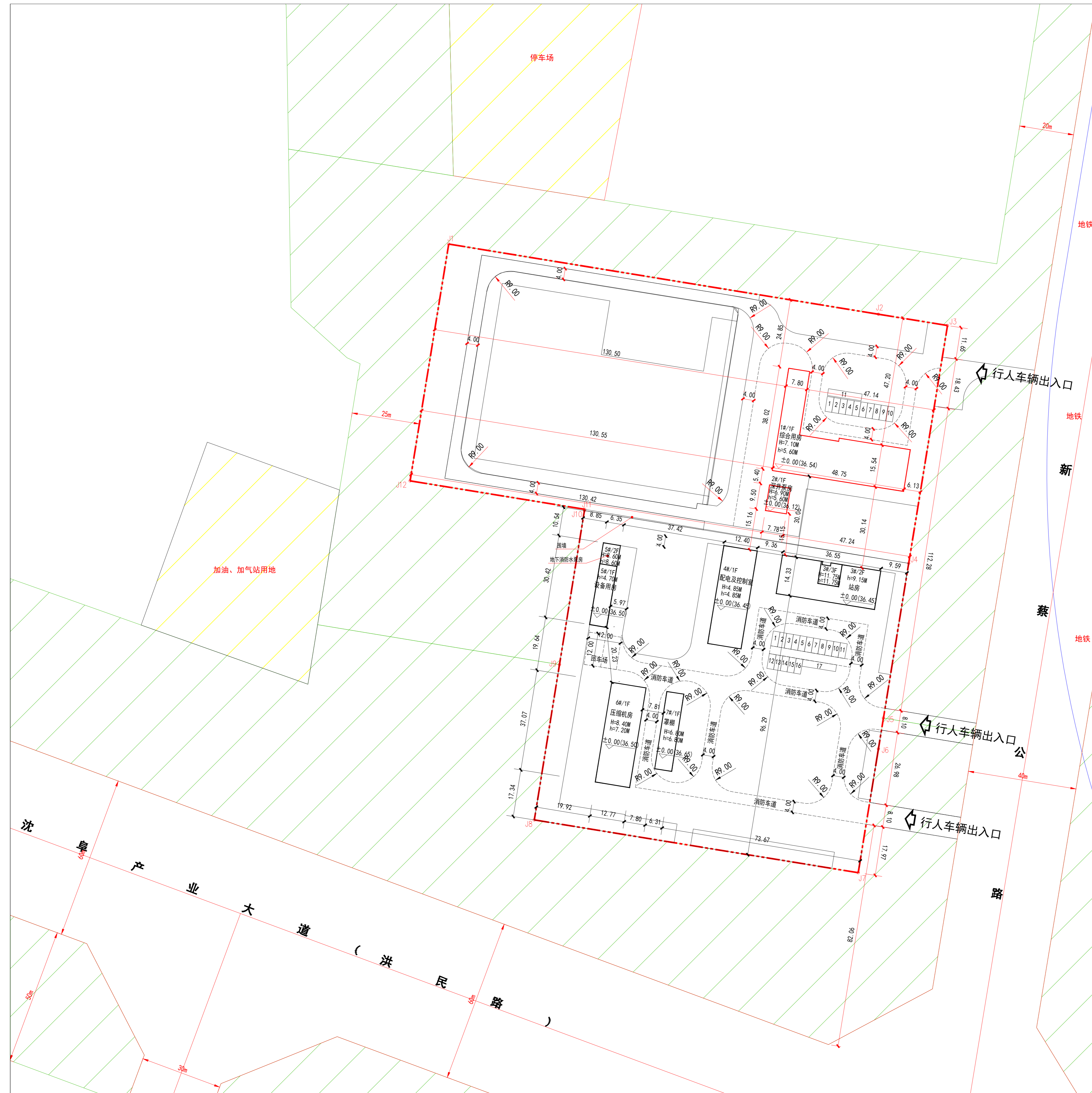
规划总平面图
