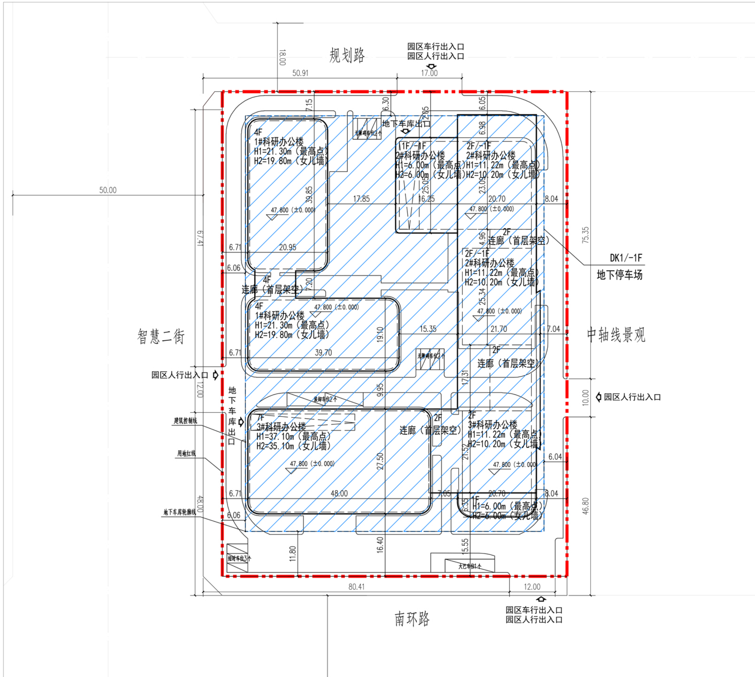
规划设计方案总平面图
