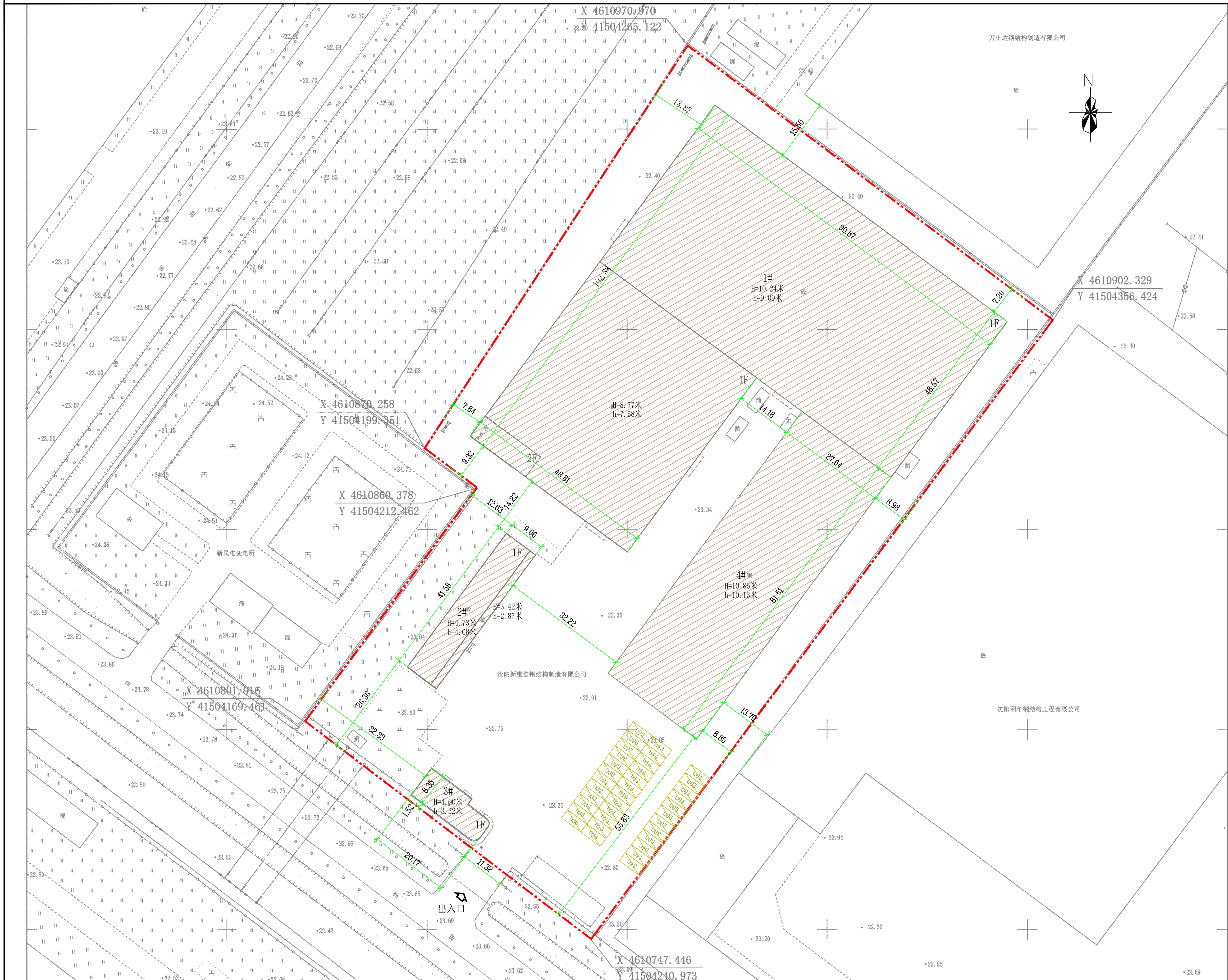
规划设计方案总平面图
