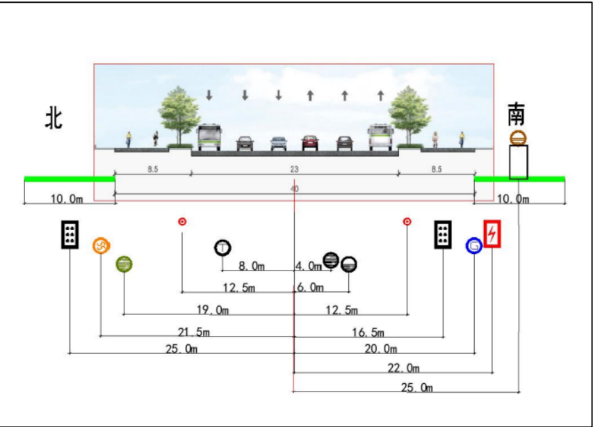
沈西一中路（细河十三北街-四环路）管线综合断面图
