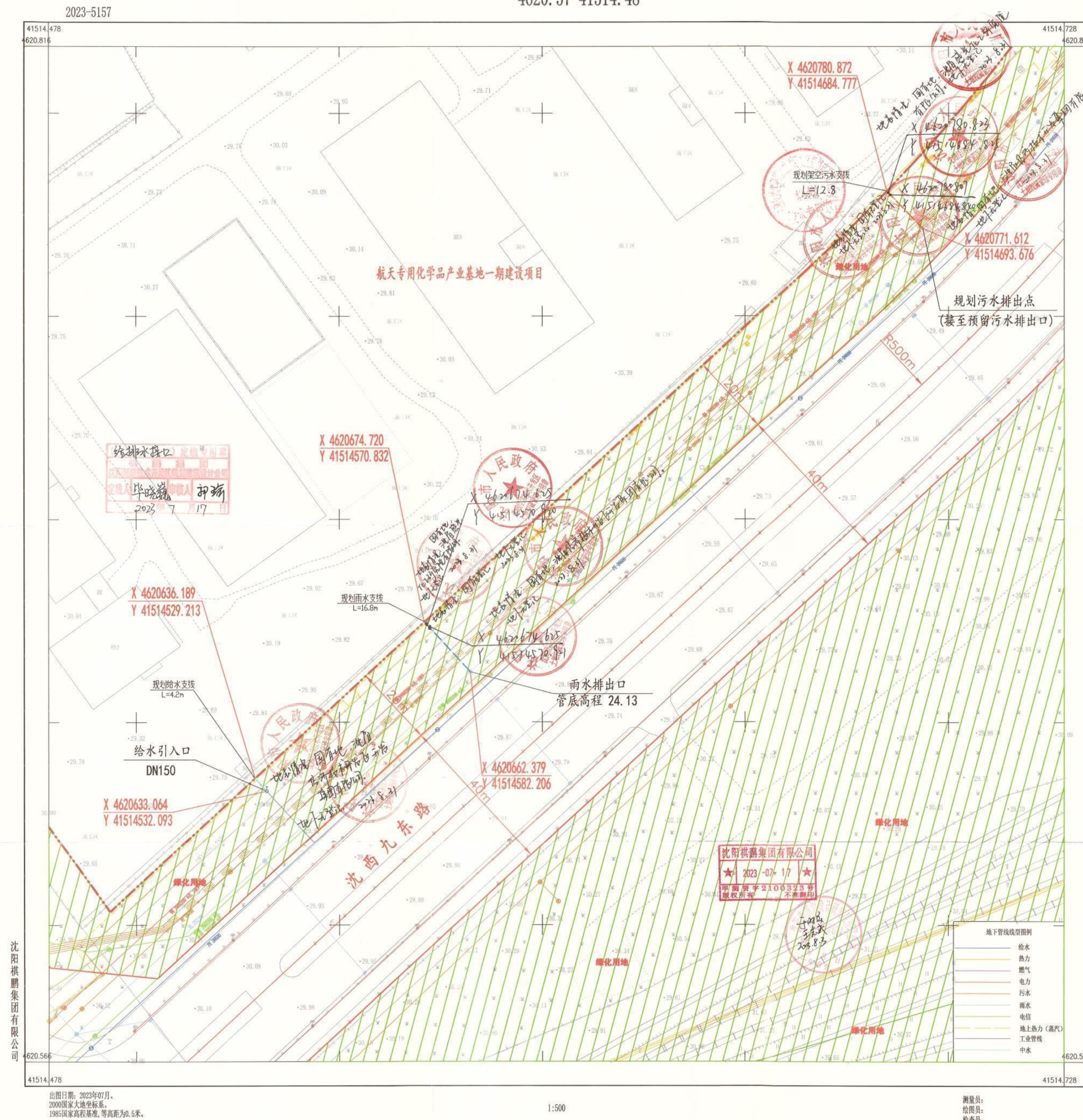
沈阳感光化工研究院有限公司市政给排水接口规划定线图 4620.57-41514.48
