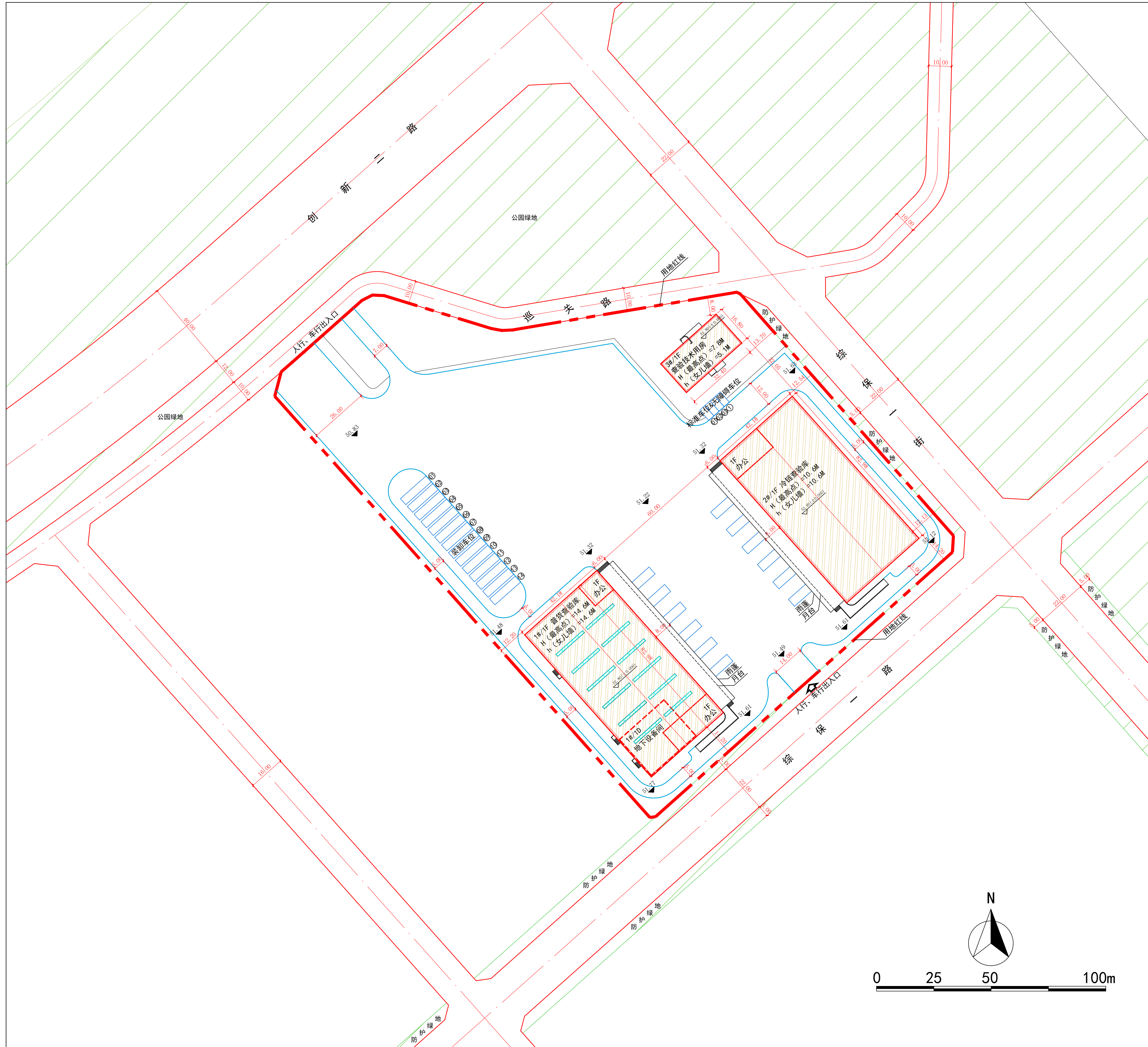
变更前总平面图
