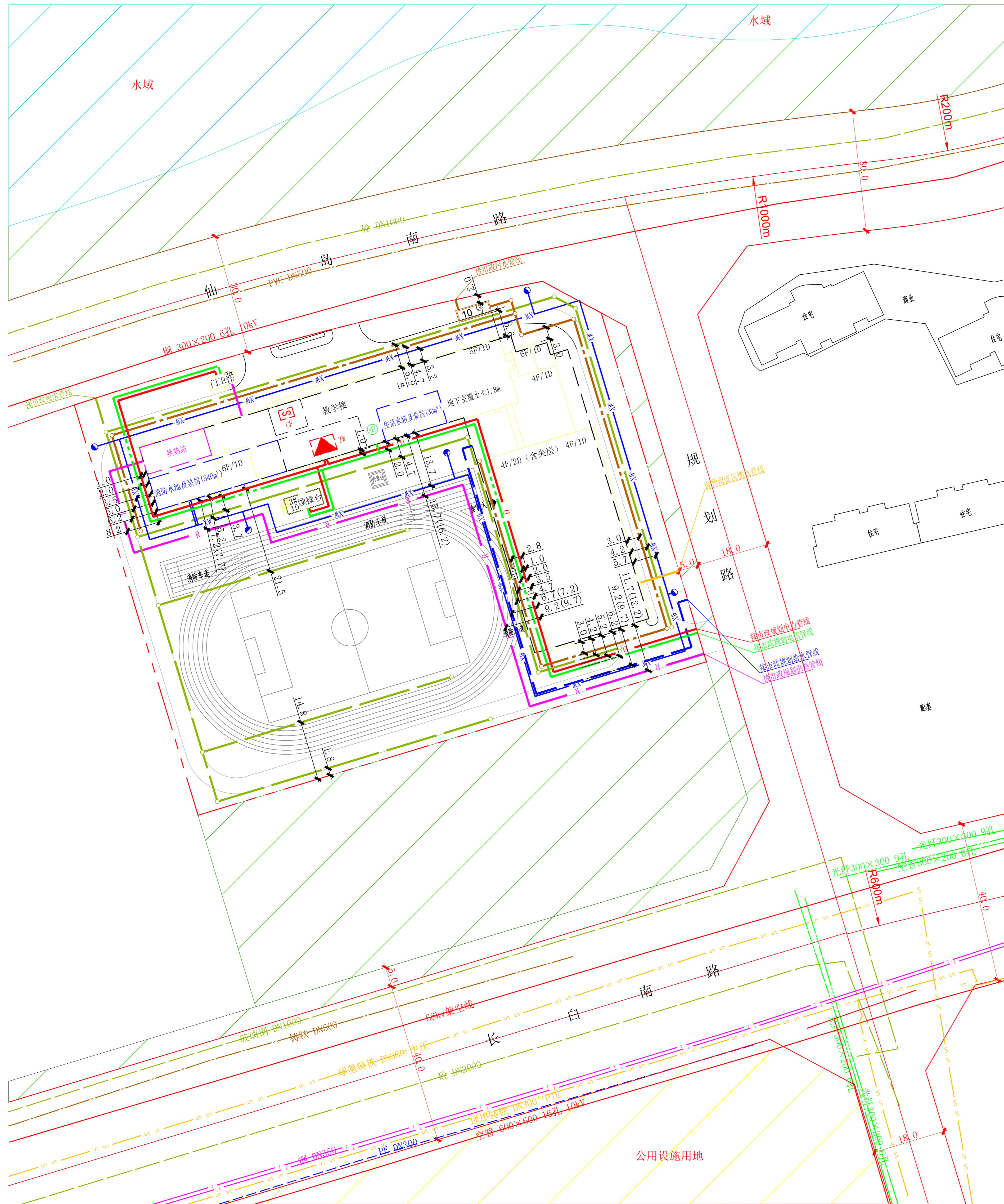
管线综合平面图1:500
