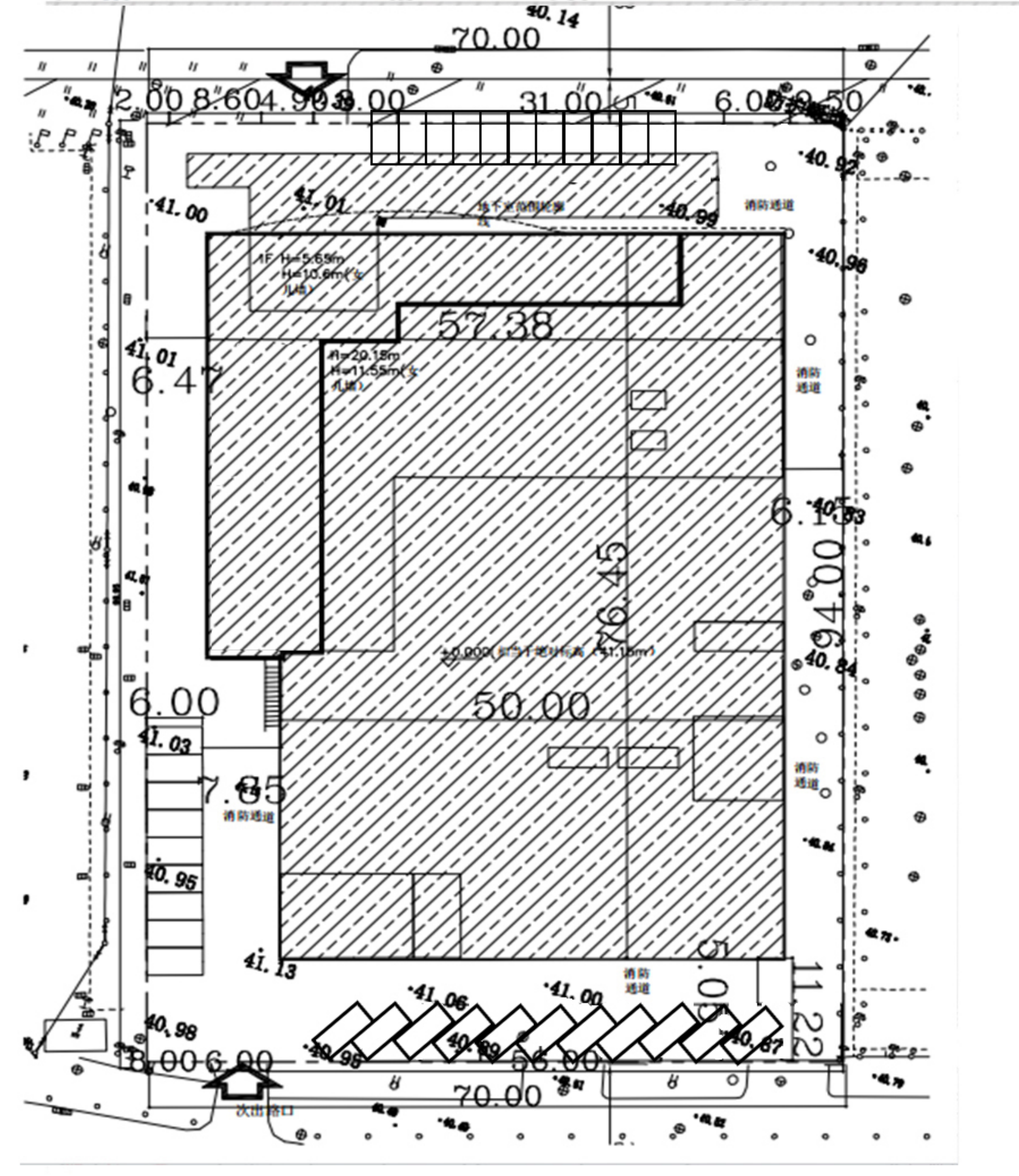
变更后总平面图
