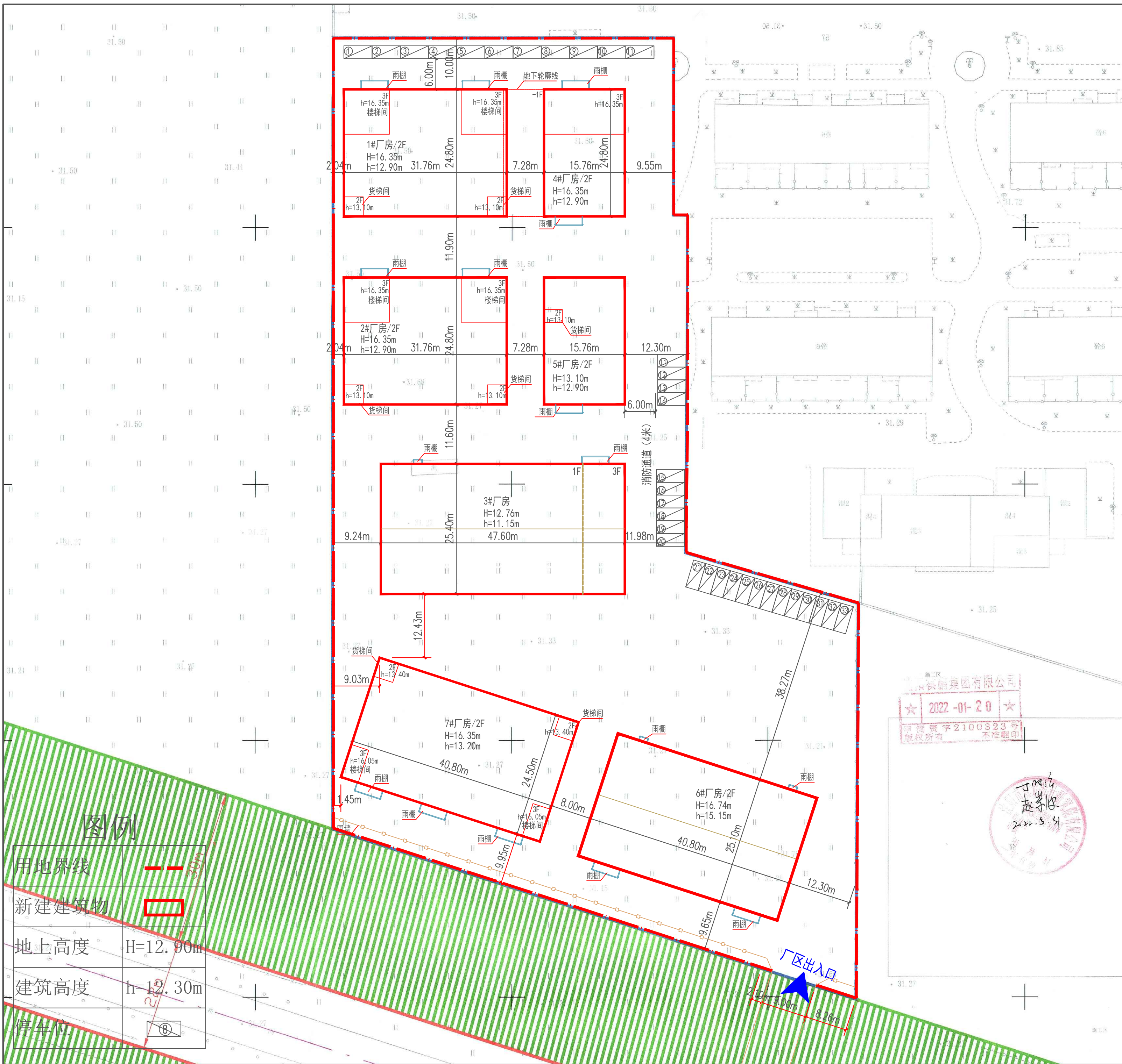
变更前总平面图
