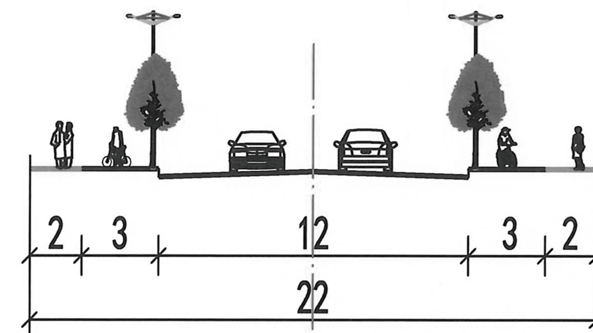
横断面布置图
