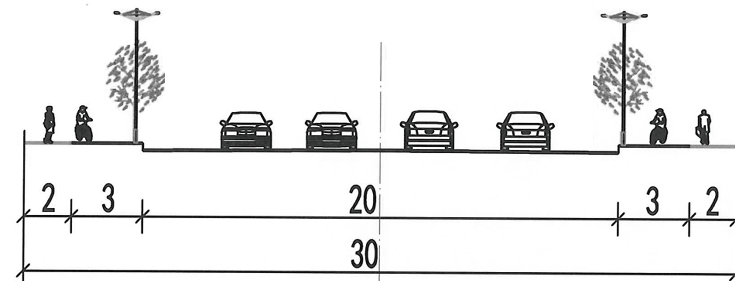
横断面布置图
