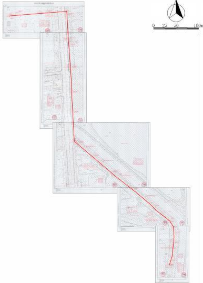
规划线位方案总平面图
