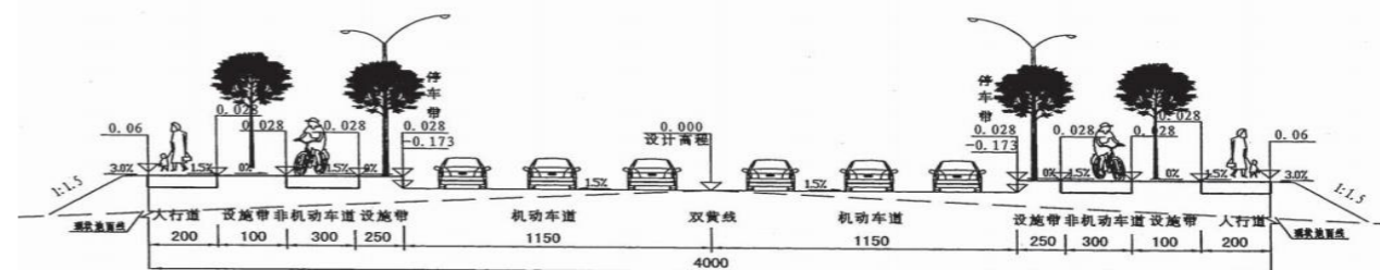
标准横断面布置图
