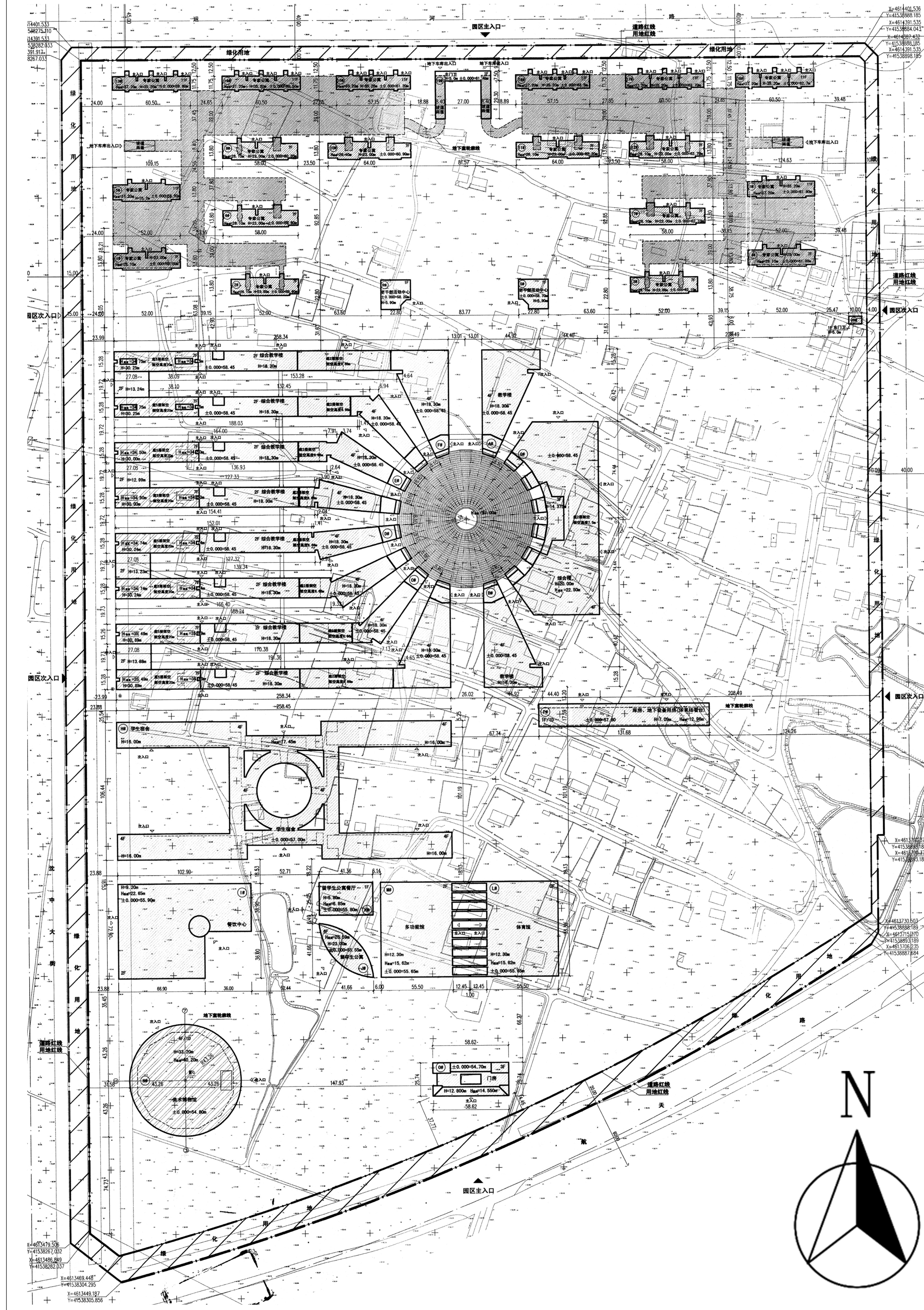
建设工程规划许可证附图
