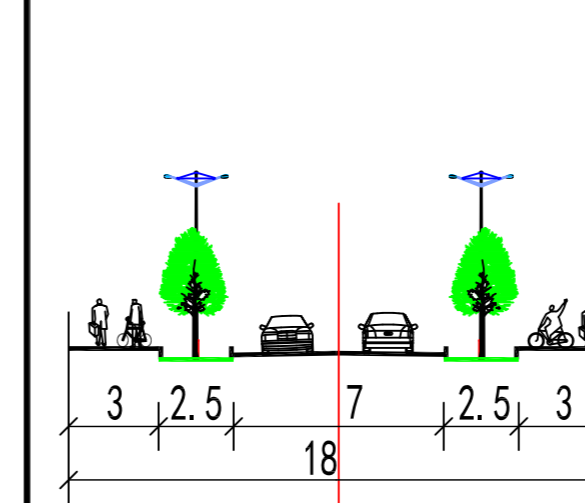
1号街道路规划横断面 (南堤东路-2号路)
