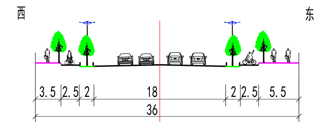
1号街道路规划横断面 (5号路-沈抚二号线)
