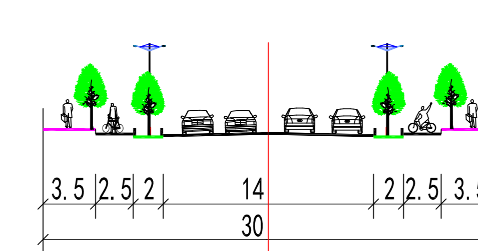
1号街道路规划横断面 (2号路-5号路)
