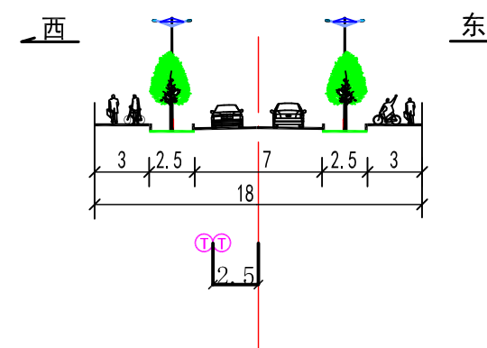
白塔西街（新运河路—永盛路） 规划横断面
