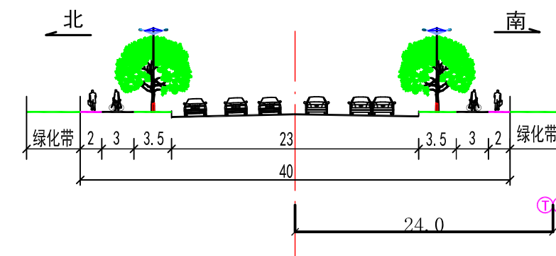
永盛路规划横断面
