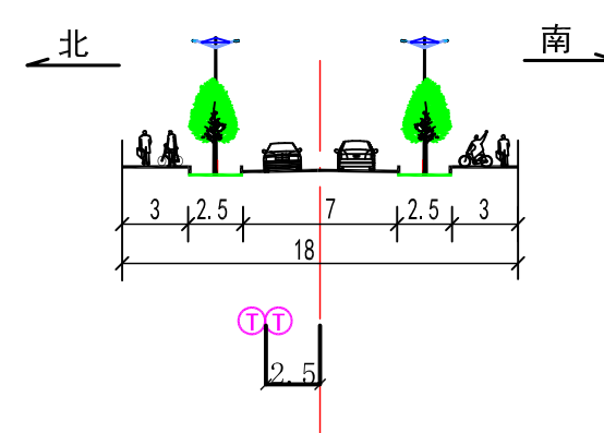
永盛路规划横断面
