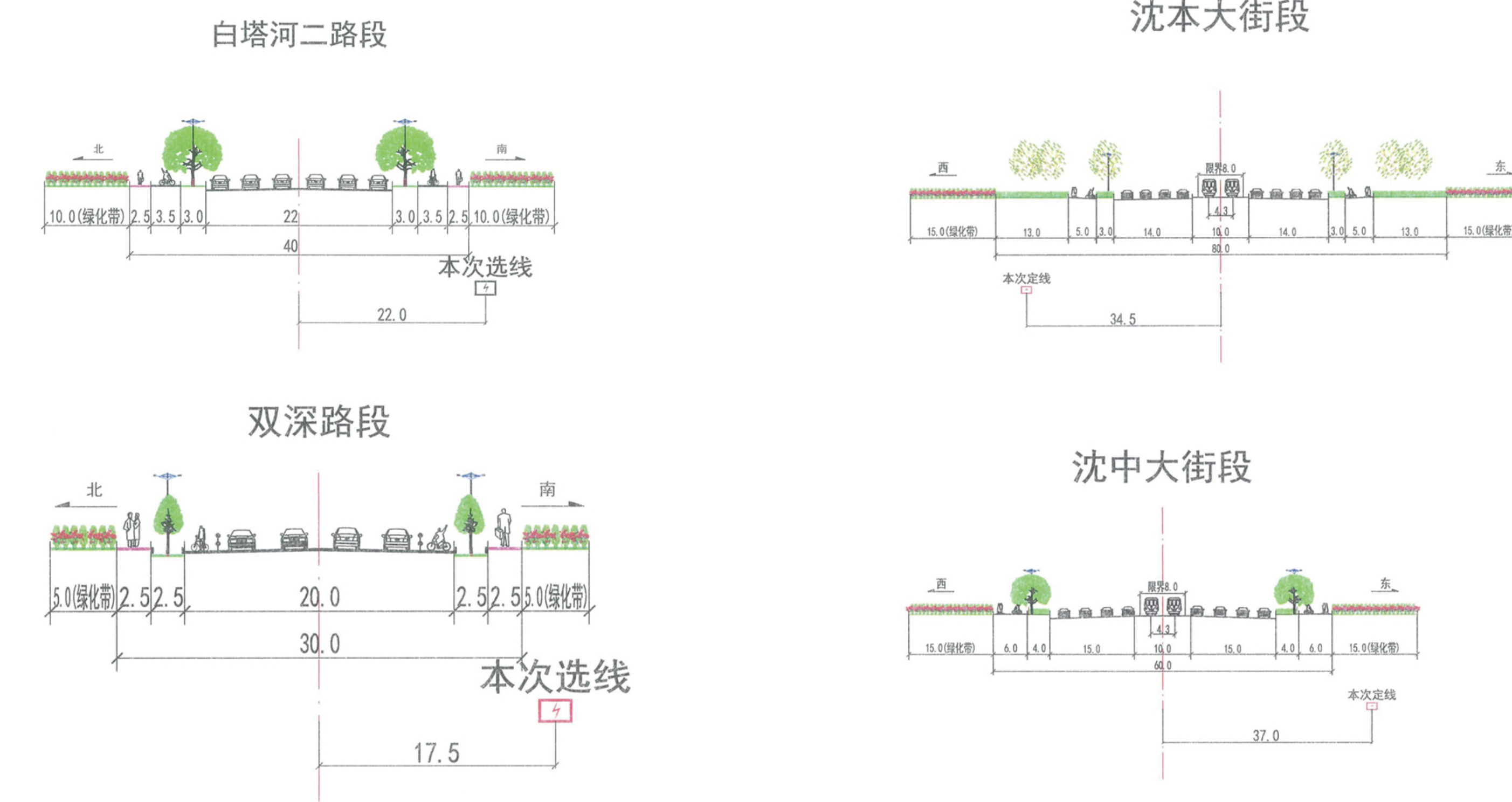
道路管线规划断面图
