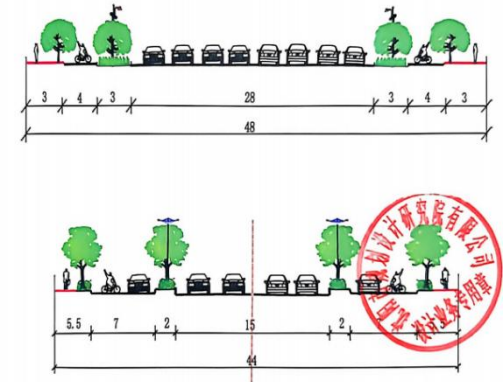
联合路道路规划横断面
