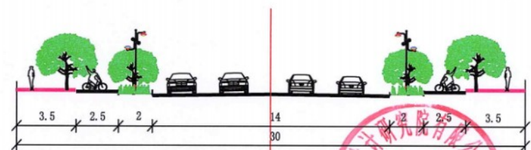
通航西街道路规划横断面
