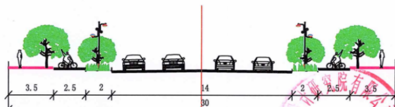
军机园7号路道路规划横断面
