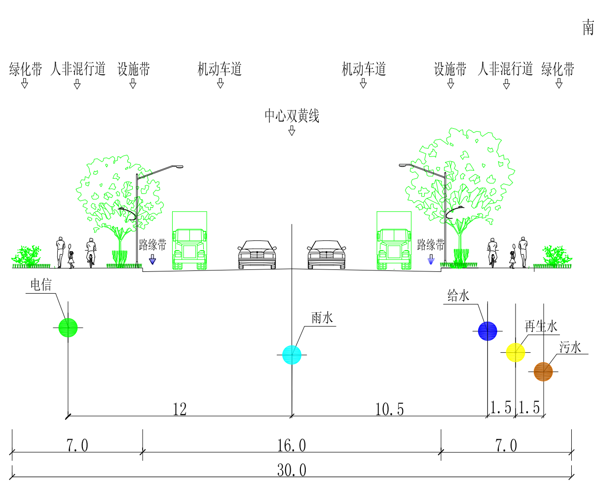
纺织园五号路管线断面示意图(八新线-绿能五路段)
