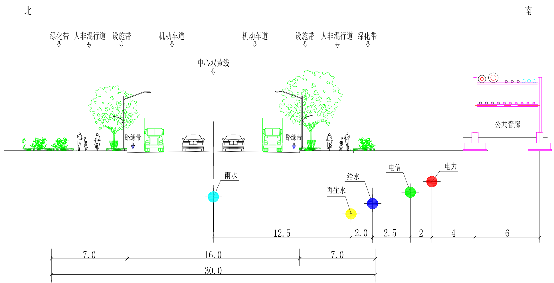
绿能大街管线断面示意图(八新线-绿能五路段)
