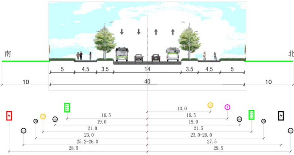
开发北六号路（四环-细河一北街西侧）电信项目 综合断面图
