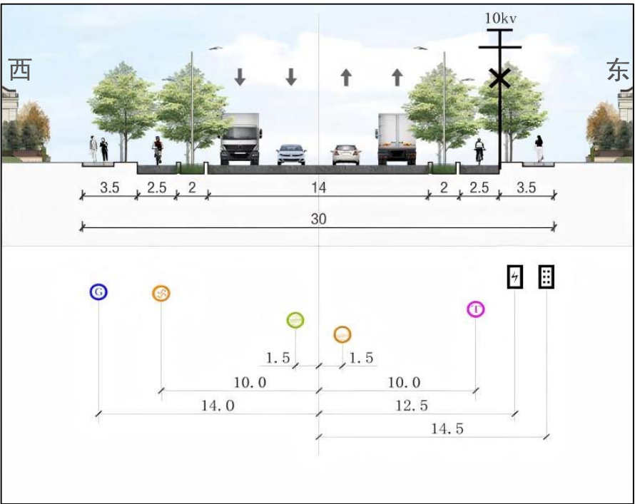
浑河三街（开发十八号路-开发十九号路）电信项目 综合断面图
