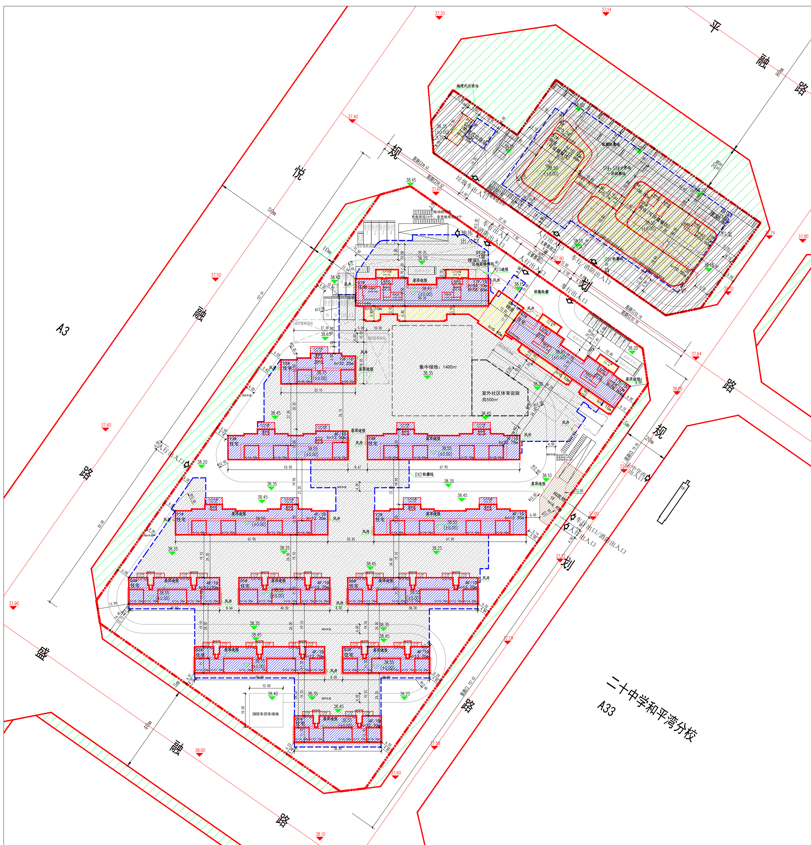
02地块规划设计方案总平面图
