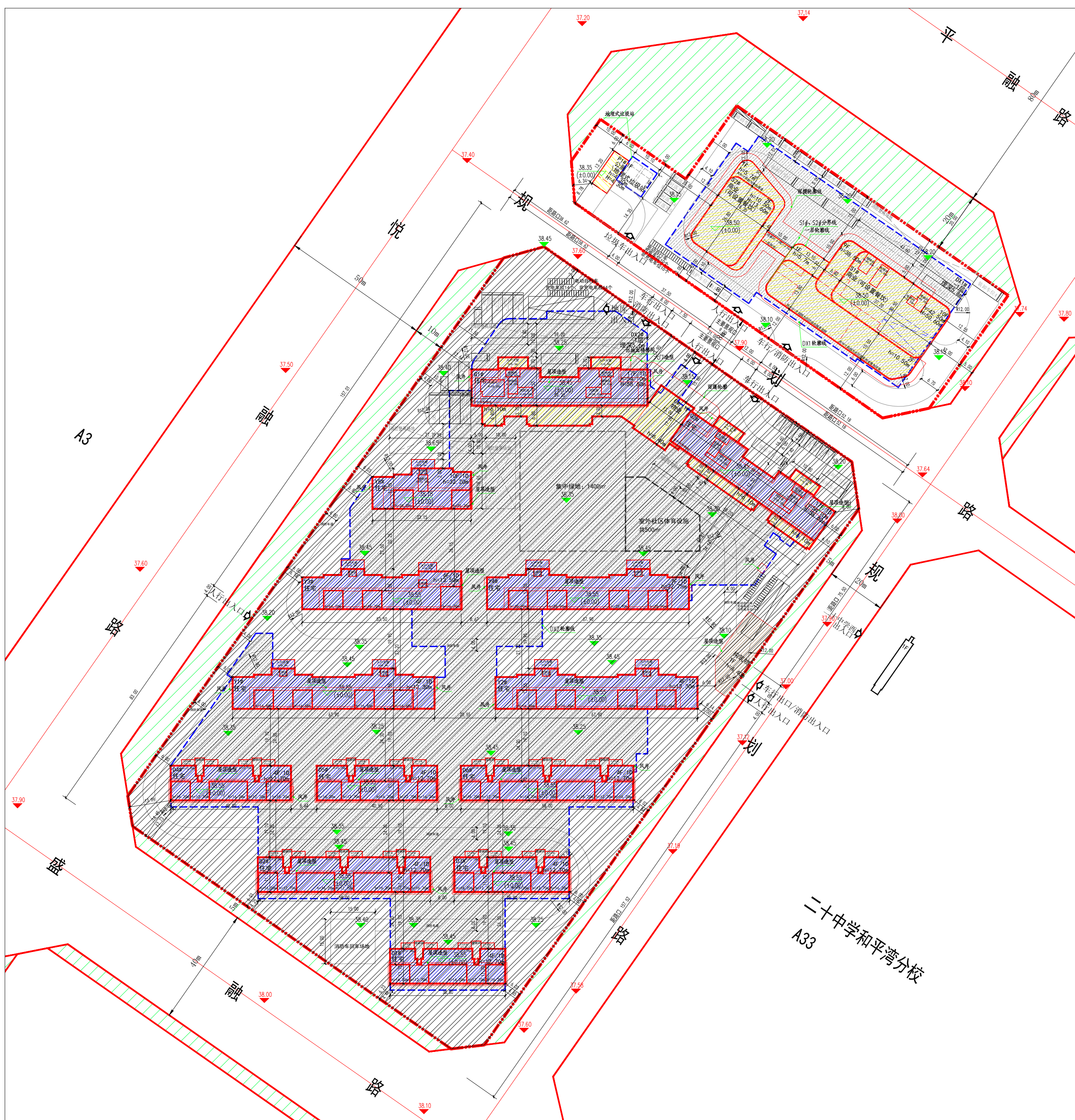
01地块规划设计方案总平面图
